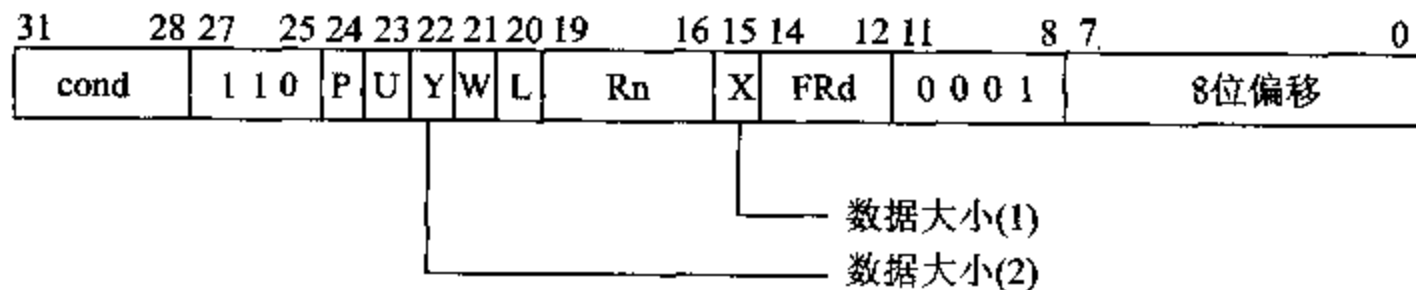
图 6.7 Load 和 Store 浮点数的二进制编码
