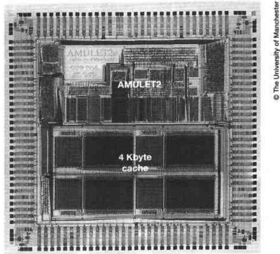
图 14.8 AMULET2e 的管芯图
