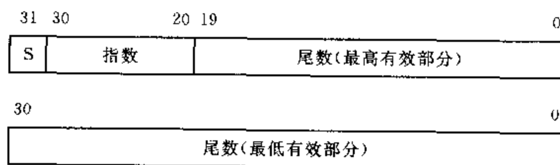
图 6.3 IEEE 754 双精度浮点数格式
