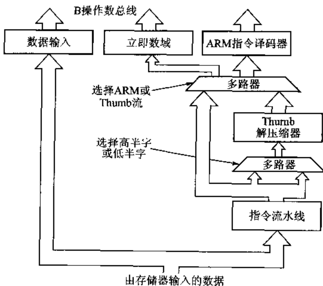
图 7.8 Thumb 指令扩展逻辑组织
