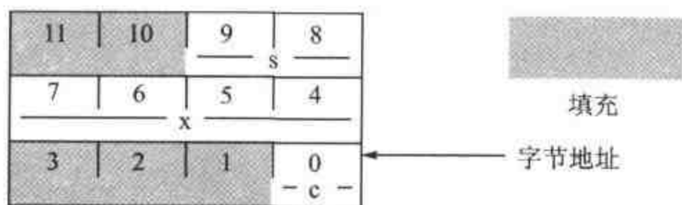
图 6.15 一般结构体存储器分配的例子
