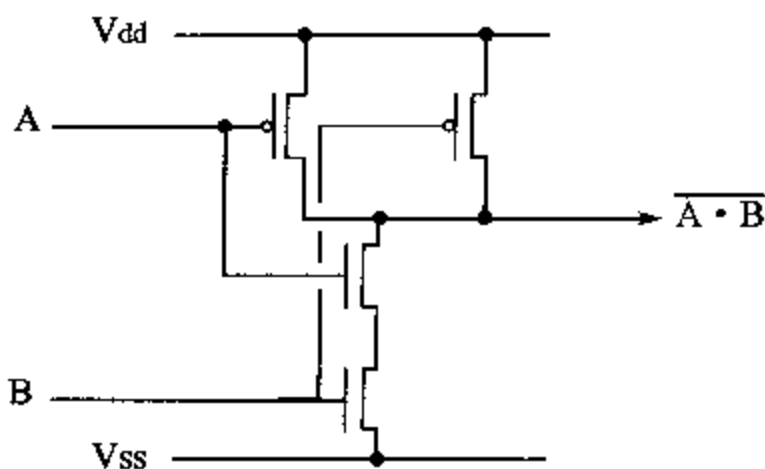
图 1.2 静态 2 输入 CMOS 与非门的晶体管电路图
