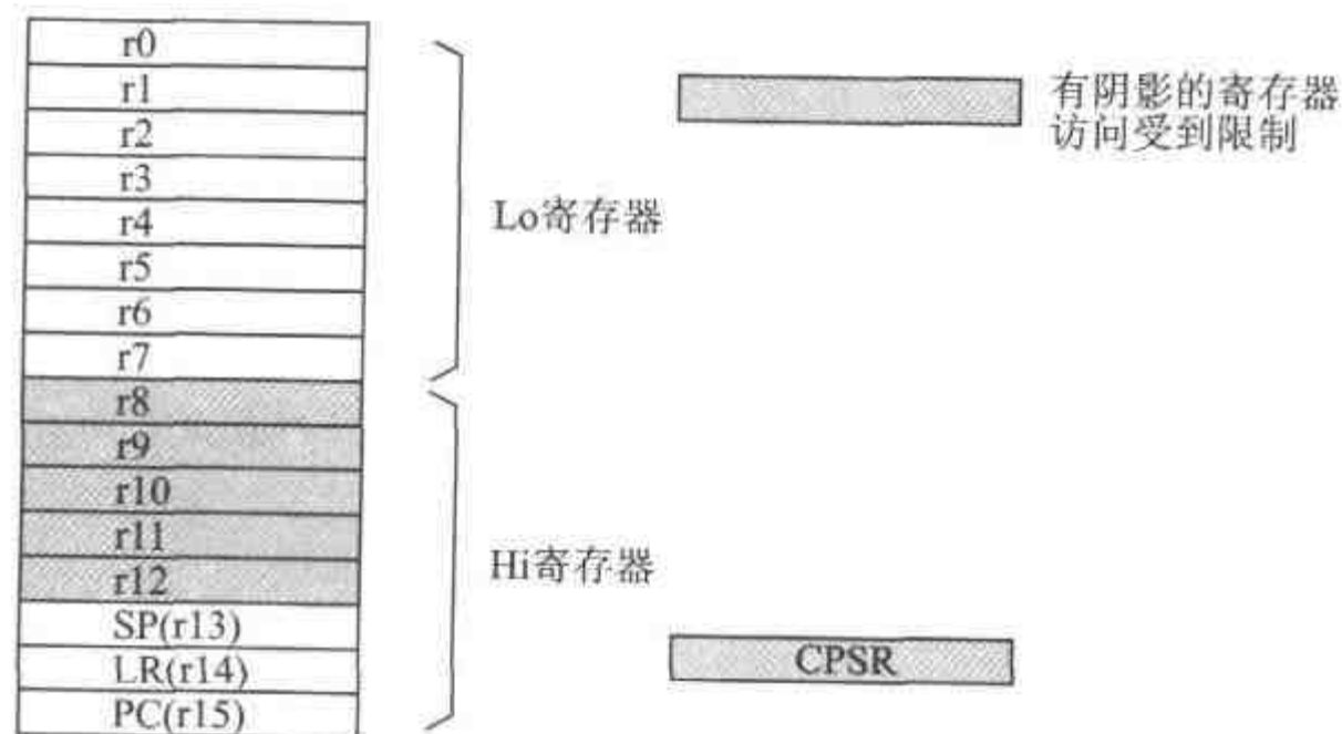
图 7.1 Thumb 指令可访问的寄存器
