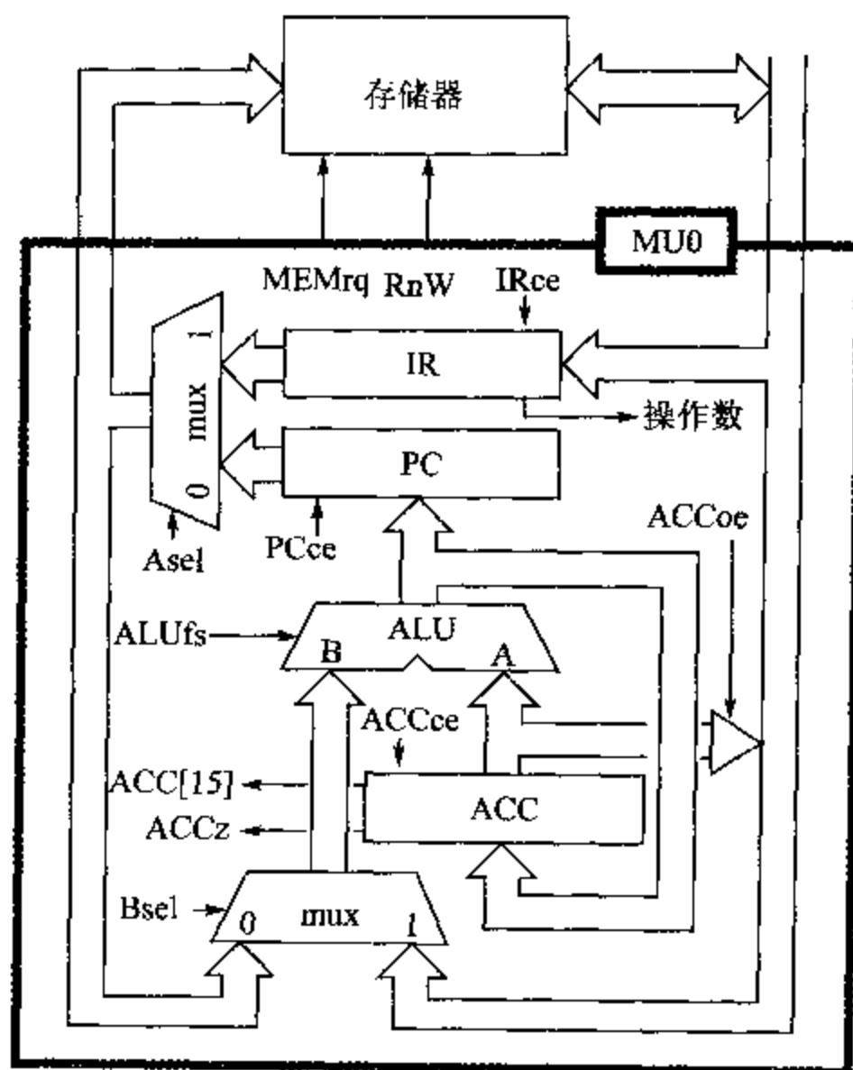
图 1.6 MU0 寄存器传输级组织
