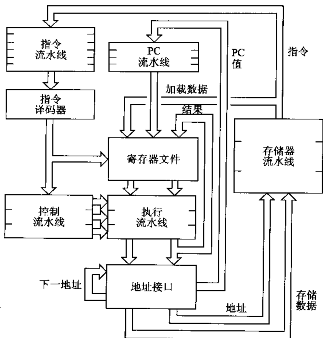
图 14.3 AMULET1 的内部组织
