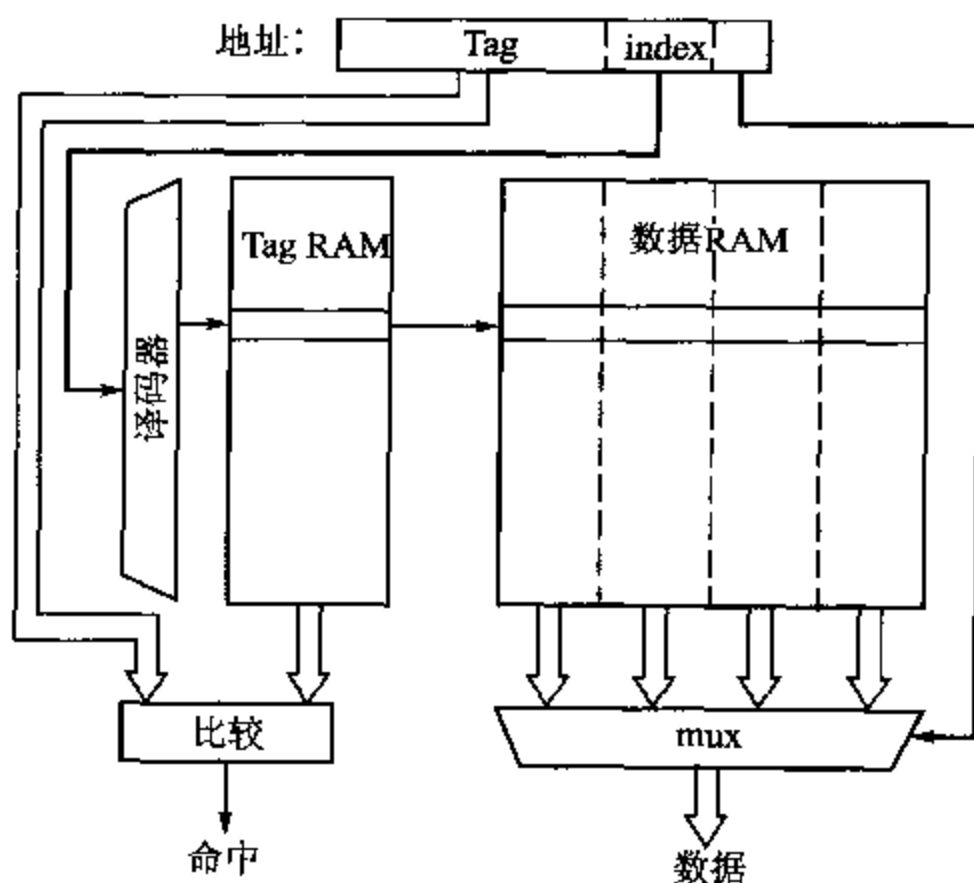
图 10.3 直接映射 Cache 组织
