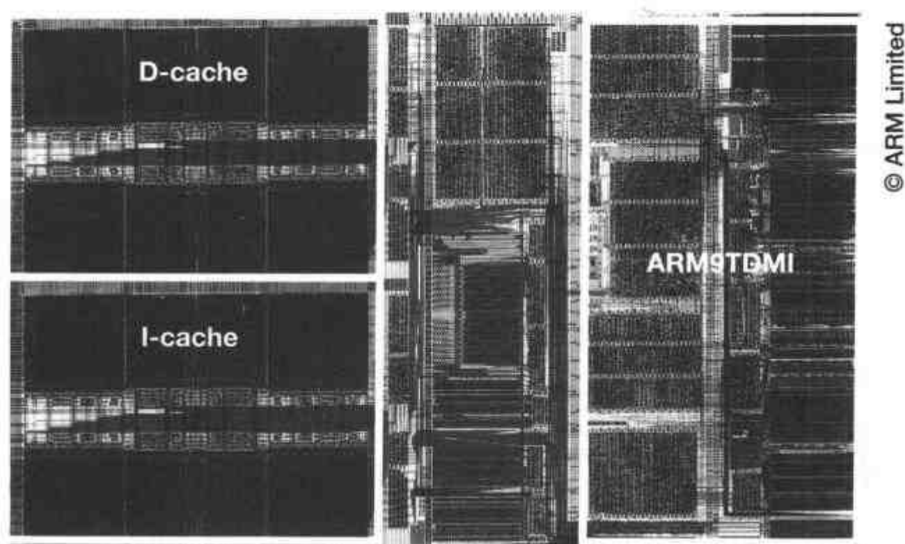
图 12.13 ARM940T CPU 版图
