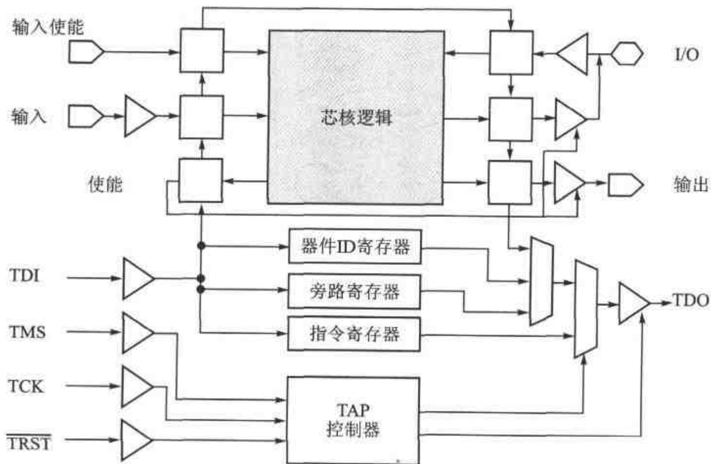
图 8.14 JTAG 边界扫描结构
