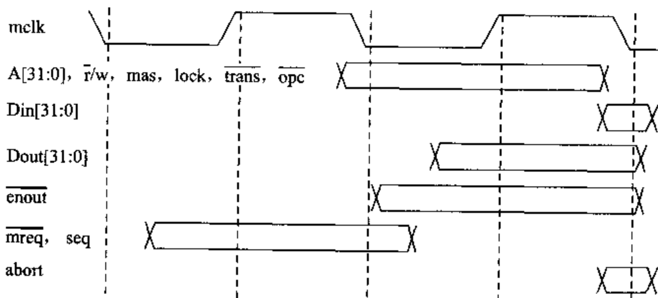
图 9.3 ARM7TDMI 核存储器和 MMU 接口时序
