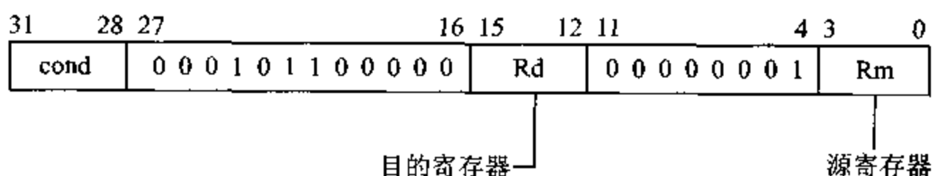
图 5.8 前导 0 计数指令的二进制编码
