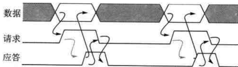
图 14.2 电平信号通信协议
