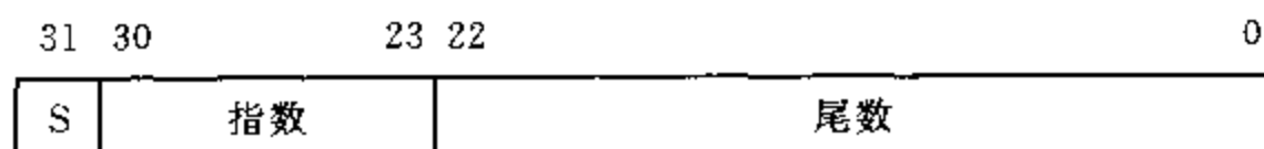
图 6.1 IEEE 754 单精度浮点数格式
