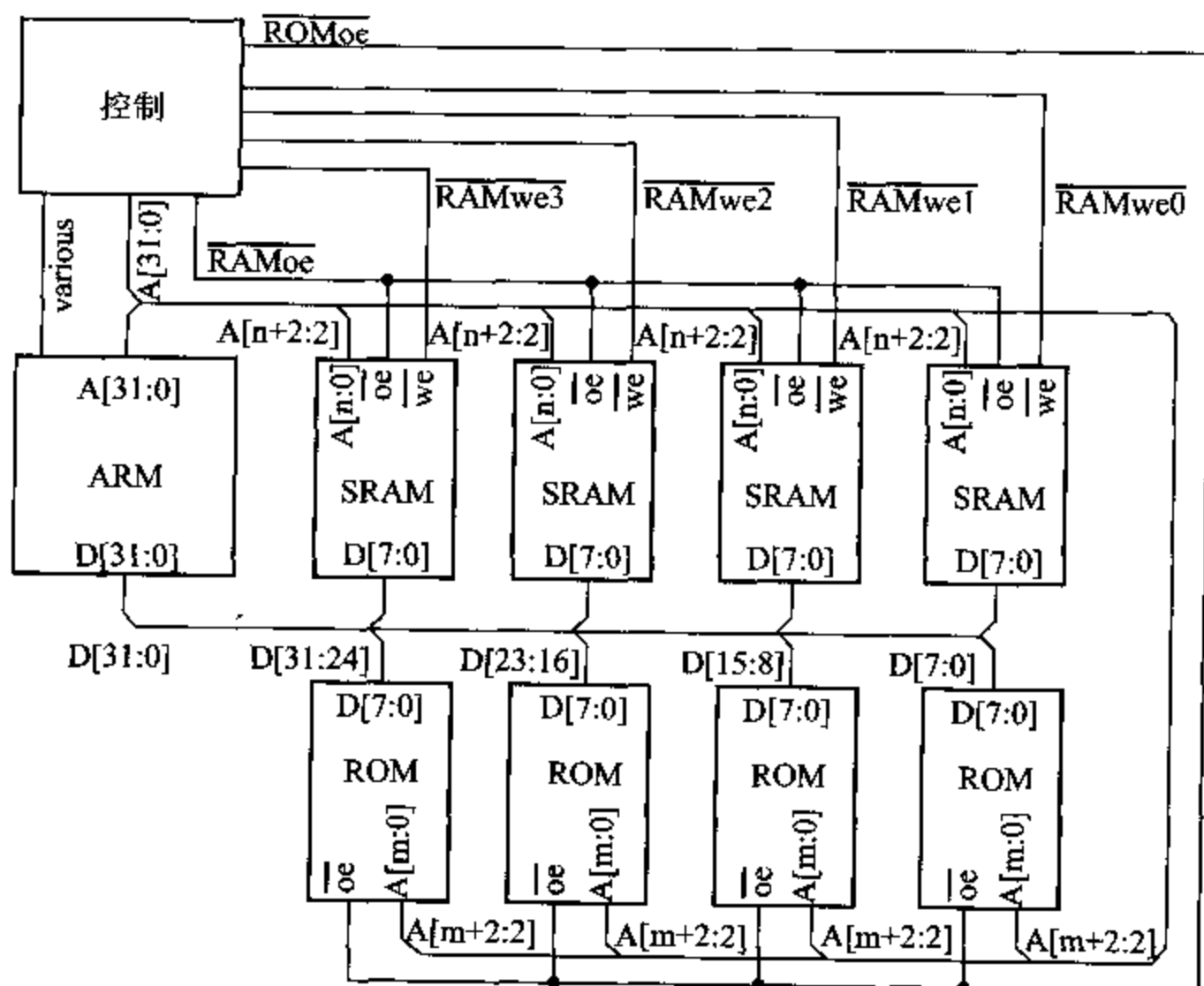
图 8.1 基本的 ARM 存储器系统
