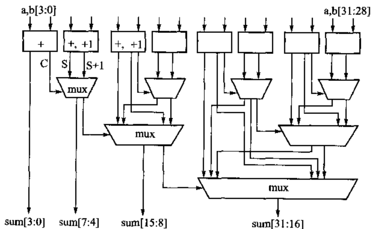
图 4.13 ARM6 的进位选择加法器方案
