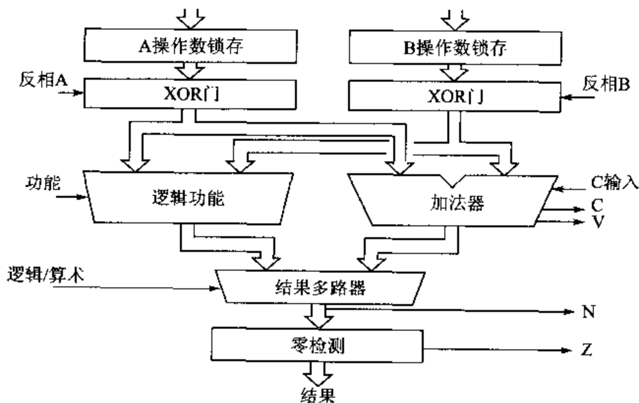
图 4.14 ARM6 中 ALU 的组织结构
