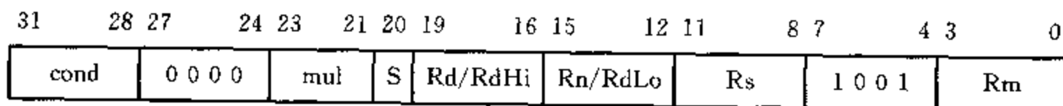
图 5.7 乘法指令的二进制编码
