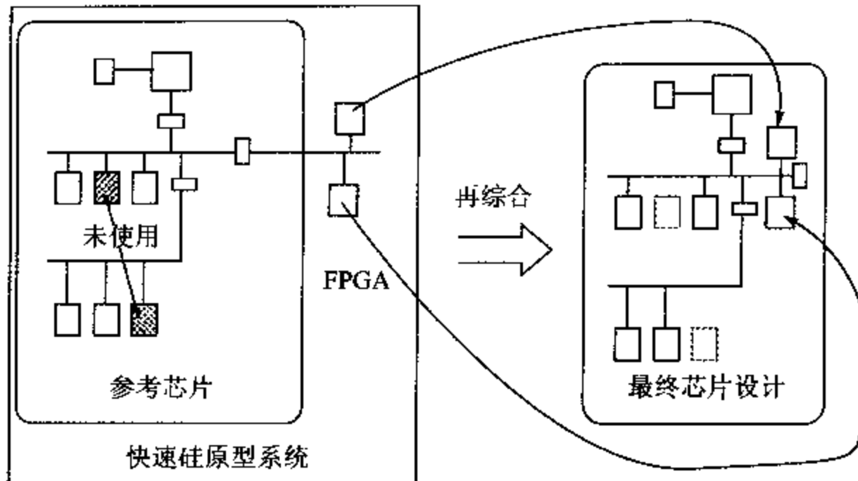
图 8.13 快速硅原型理论
