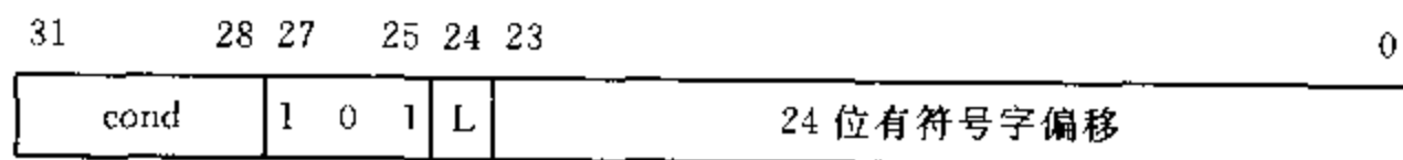
图 5.3 转移和转移链接指令的二进制编码
