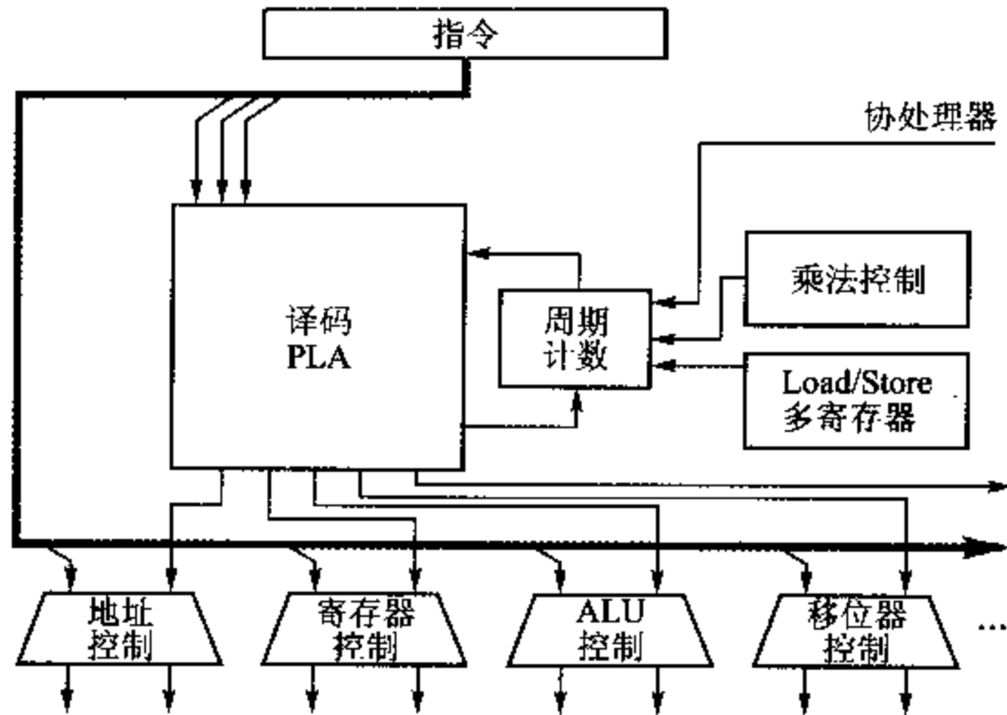
图 4.21 ARM 控制逻辑的结构
