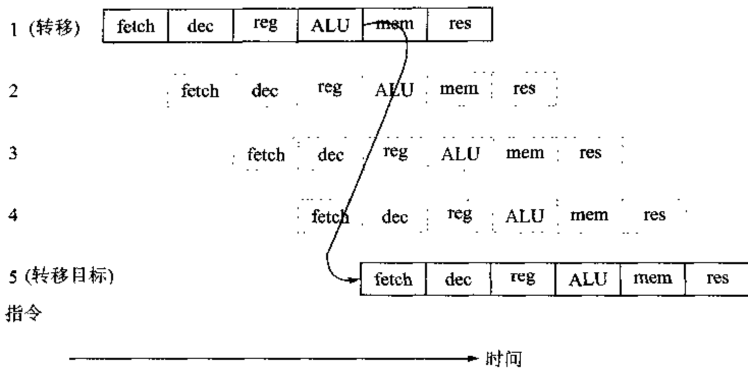
图 1.15 流水线的转移行为
