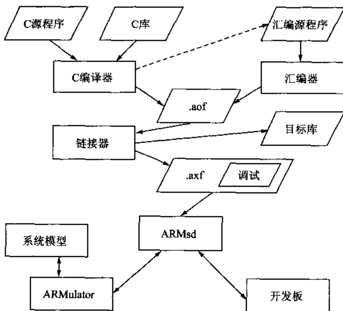
图 2.4 ARM 交叉开发工具套件的结构
