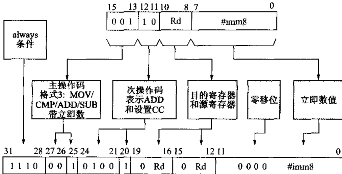
图 7.9 Thumb 到 ARM 的指令映射
