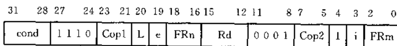
图 6.10 浮点寄存器传送二进制编码
