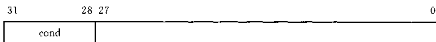
图 5.2 ARM 的条件代码域
