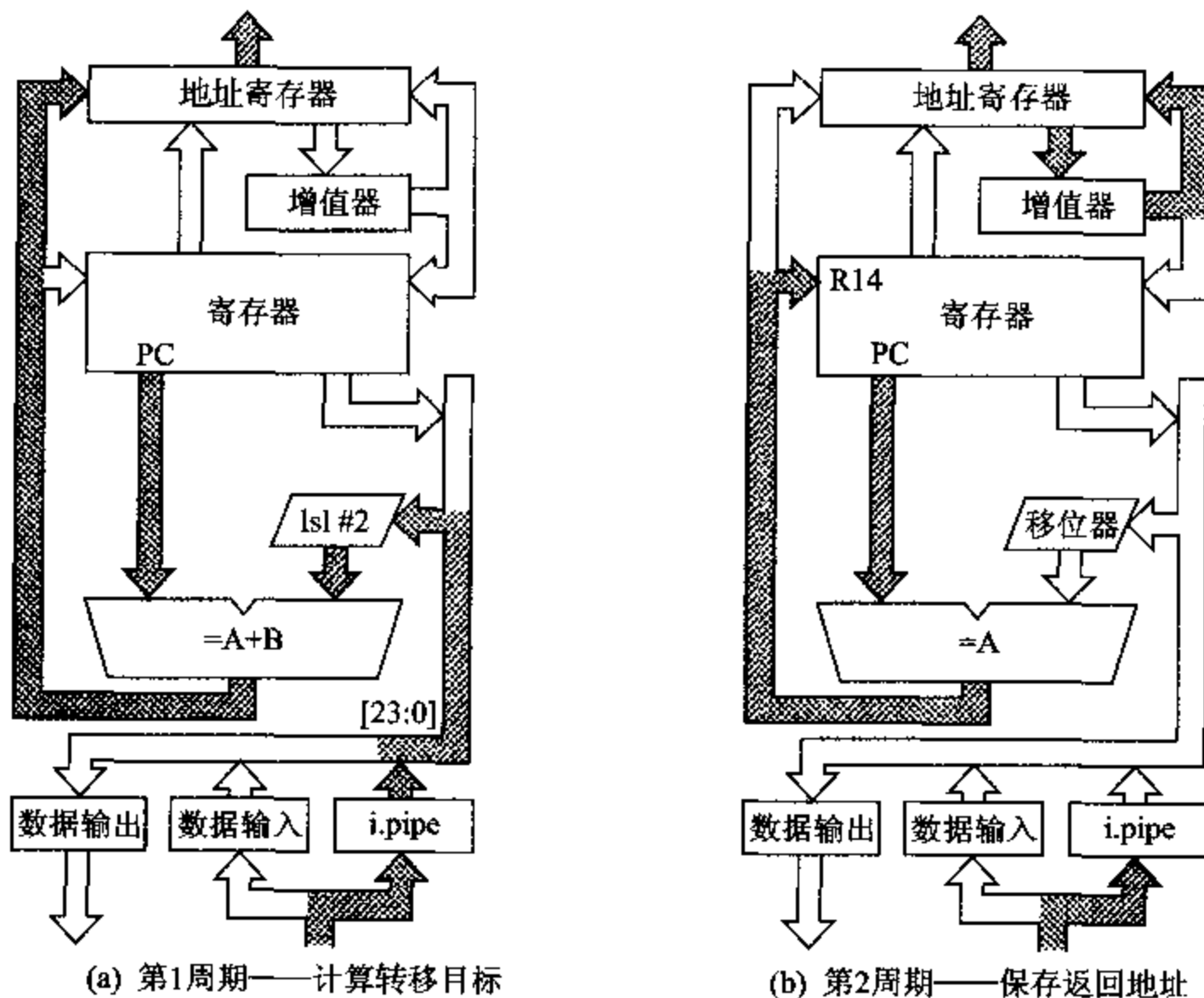
图 4.7 转移指令的 3 个周期中的前两个周期
