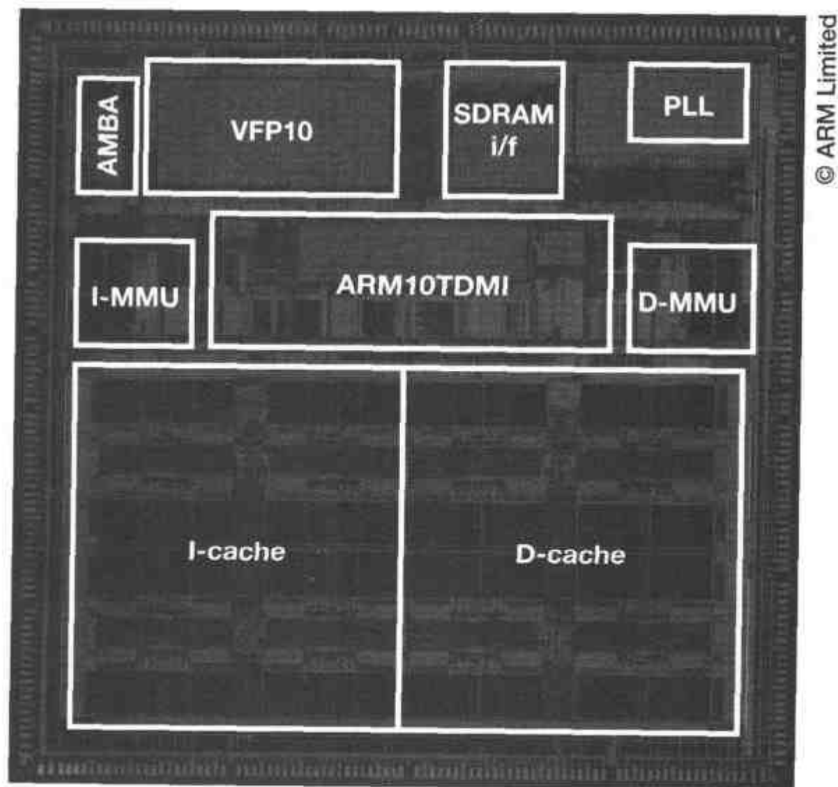
图 12.14 ARM10200 芯片版图
