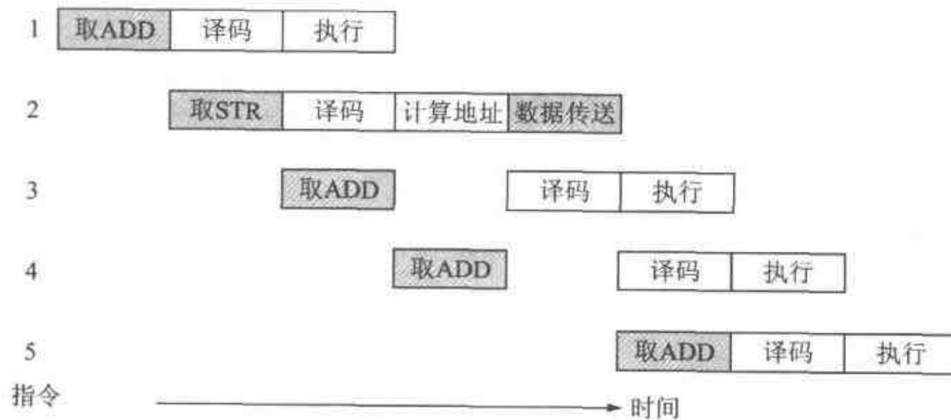
图 4.3 ARM 多周期指令的 3 级流水线操作
