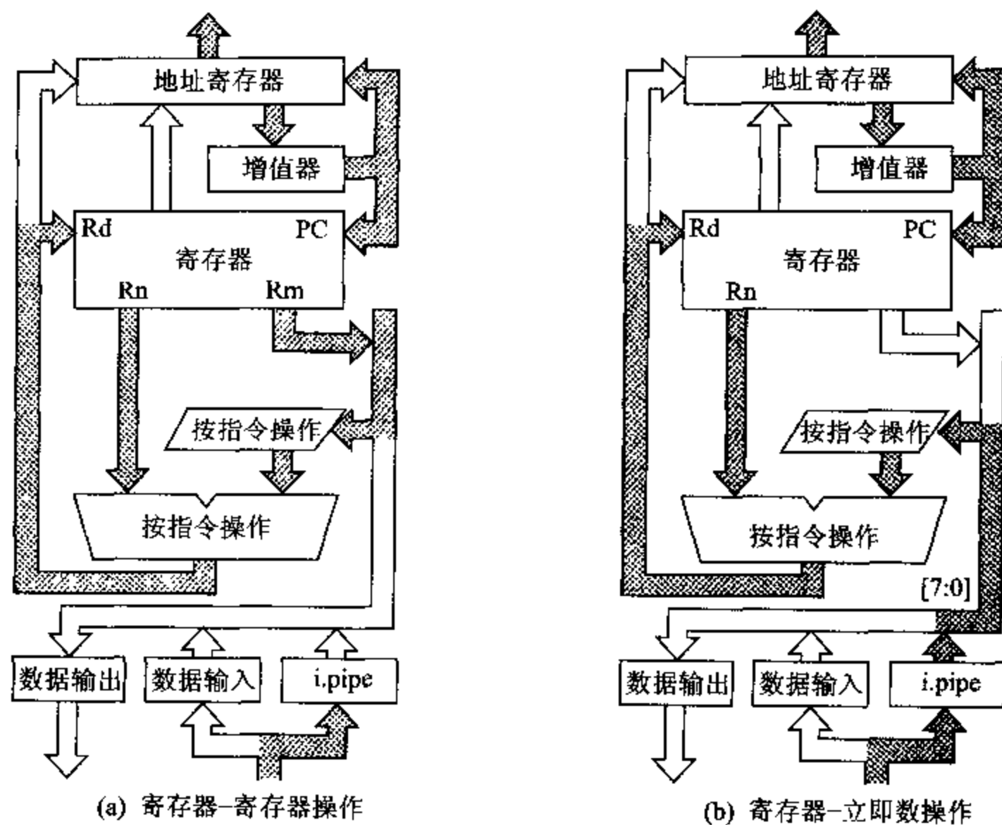
图 4.5 数据处理指令的数据通路行为
