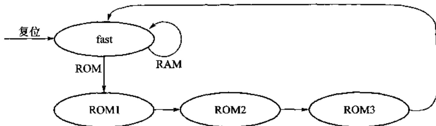
图 8.3 ROM 等待控制状态转换图
