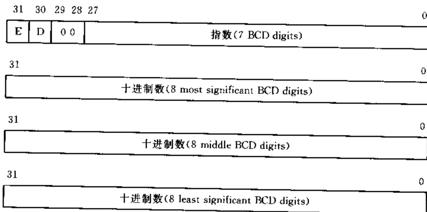
图 6.6 IEEE 754 扩展的压缩十进制浮点数格式
