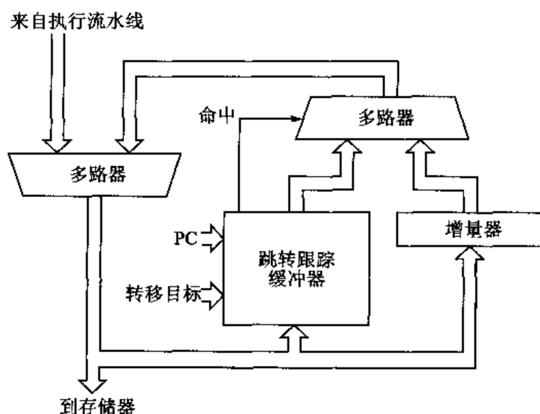
图 14.6 AMULET2 跳转跟踪缓冲器
