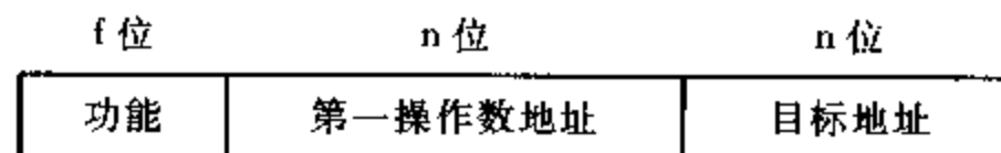
图 1.10 2 地址指令格式
