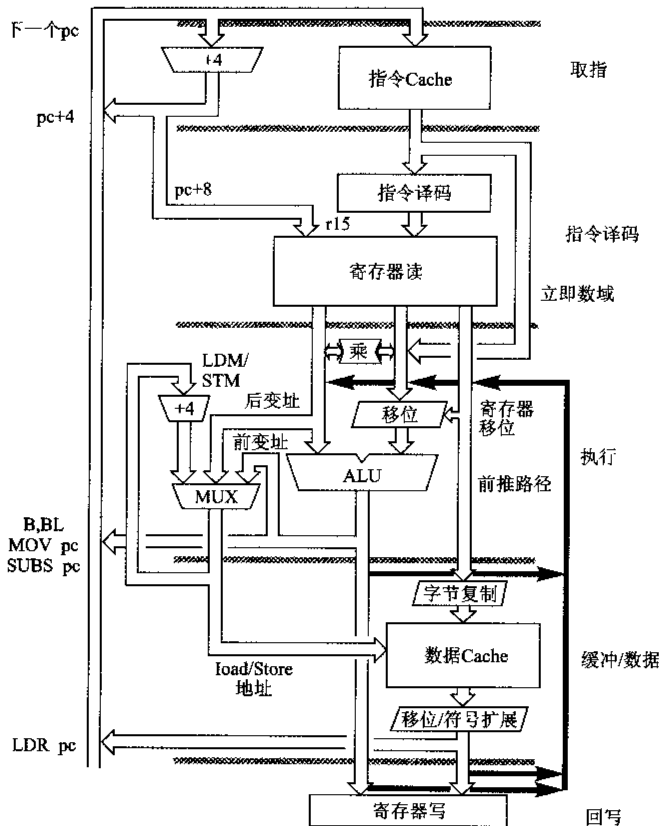
图 4.4 ARM9TDMI 5 级流水线的组织结构
