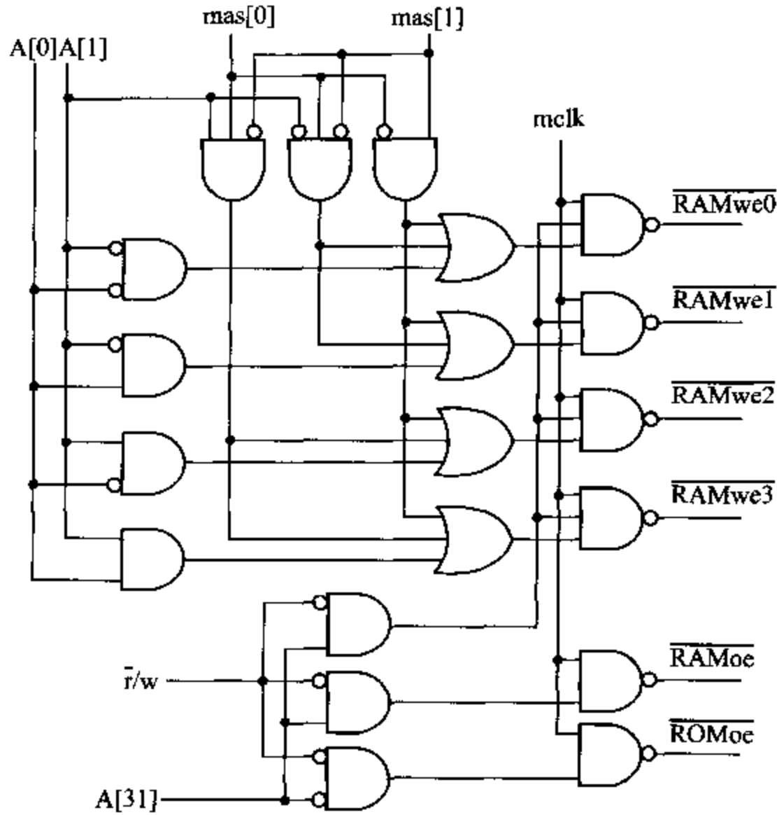
图 8.2 简单的 ARM 存储器系统控制逻辑
