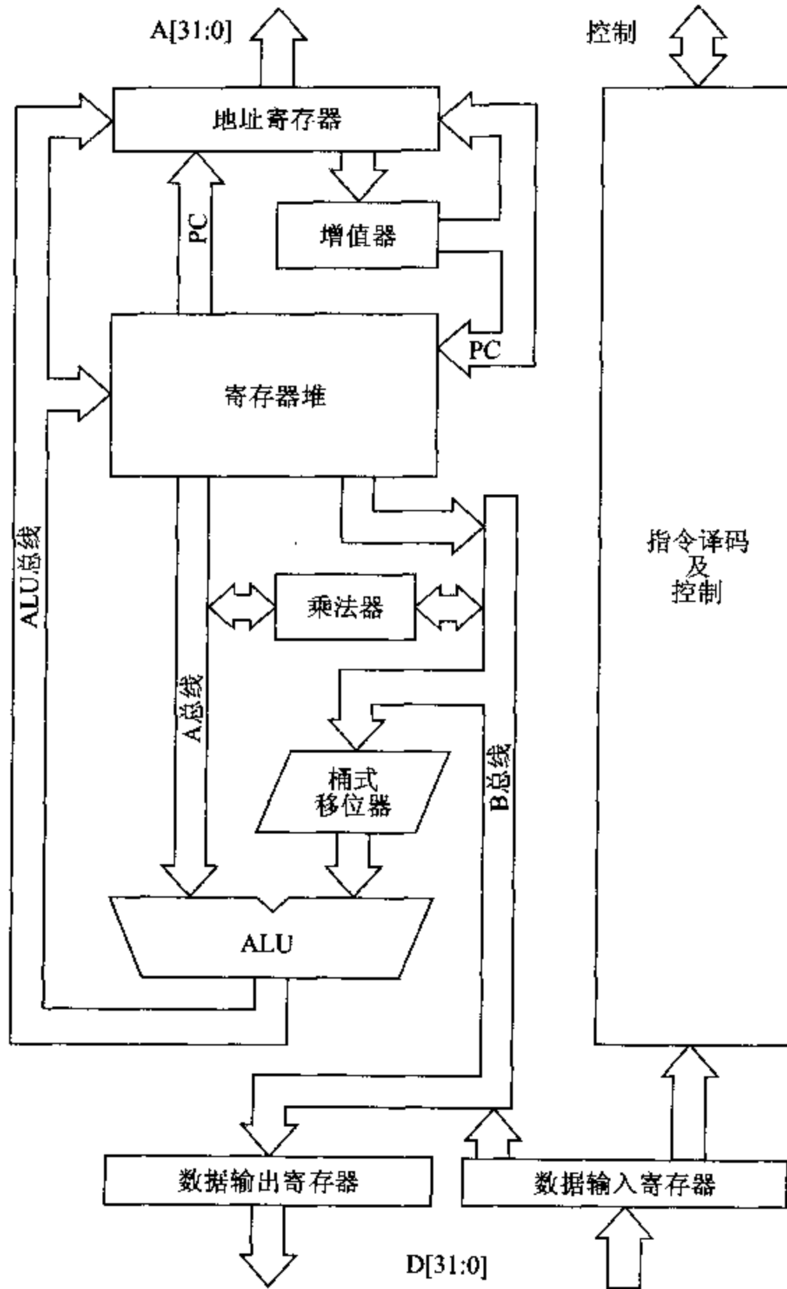
图 4.1 3级流水线 ARM 的组织
