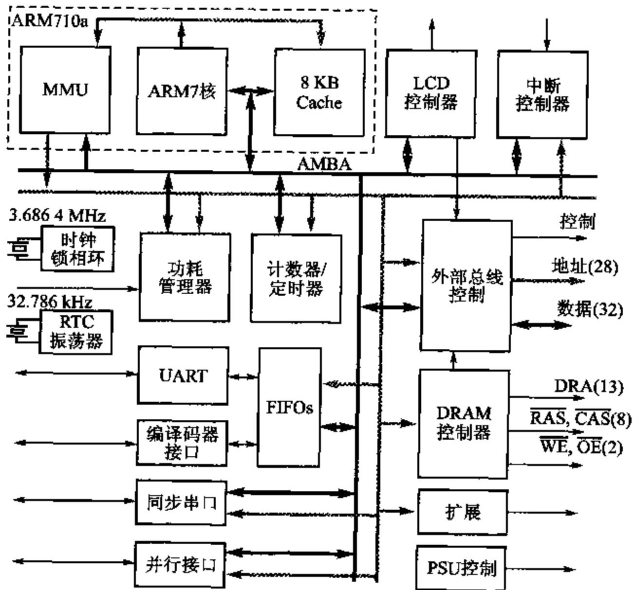
图 13.13 ARM7100 的组织结构
