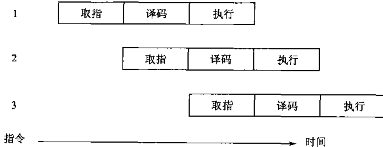
图 4.2 ARM 单周期指令的 3 级流水线操作
