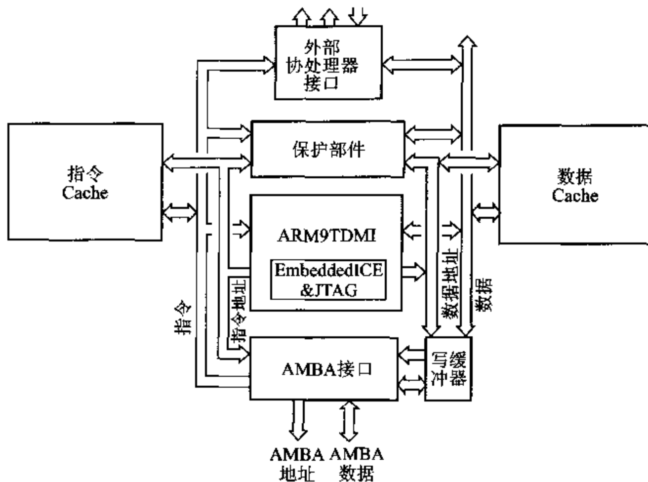
图 12.12 ARM940T 的组织
