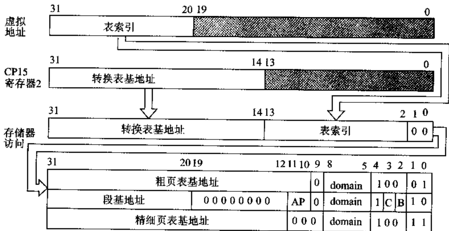
图 11.3 第一级转换的读取
