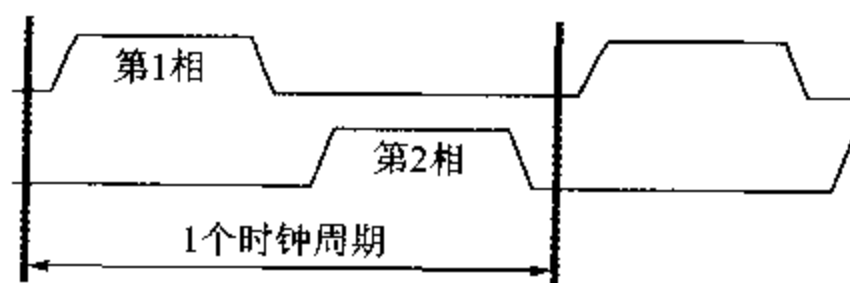
图 4.8 两相非重叠时钟方案
