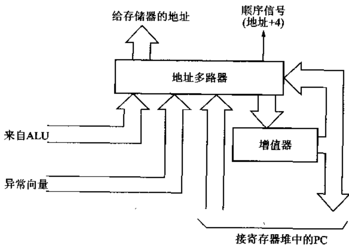
图 8.8 ARM 地址寄存器结构
