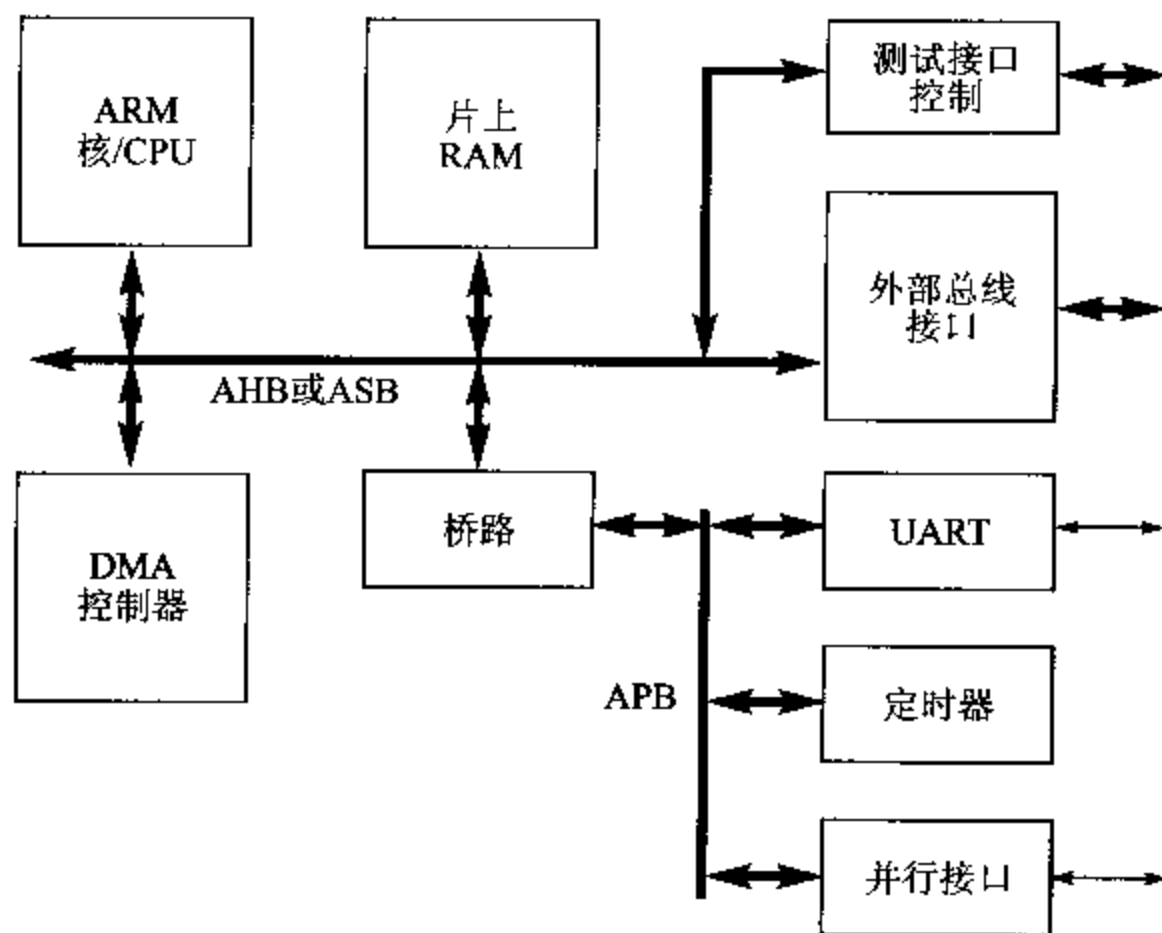
图 8.11 典型的基于 AMBA 的系统
