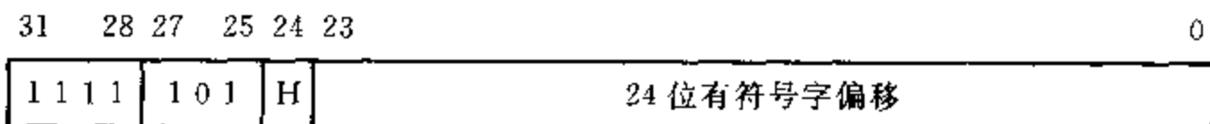
图 5.4 转移交换(带链接选项)指令的二进制编码
