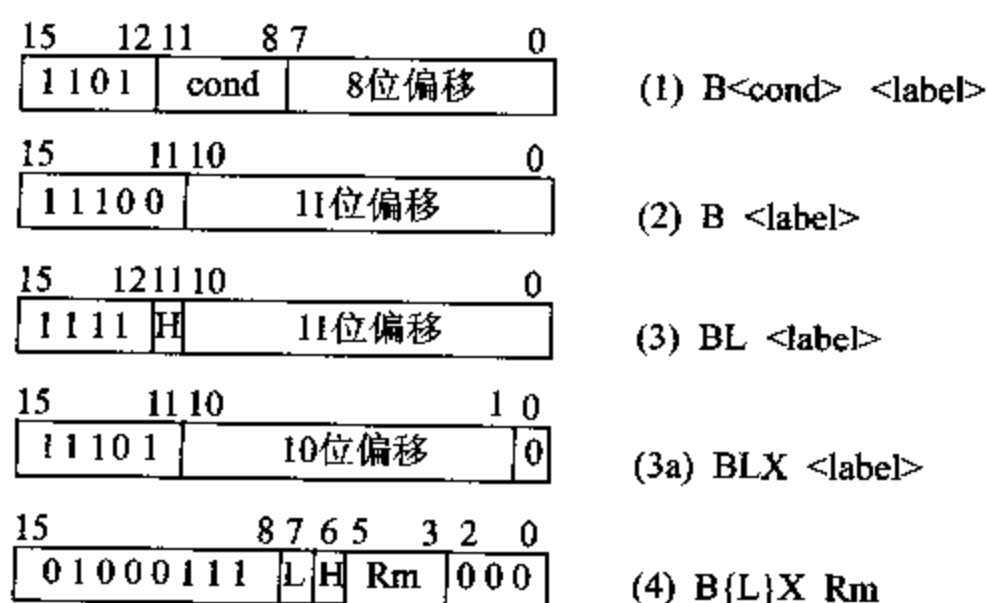
图 7.2 Thumb 转移指令二进制编码
