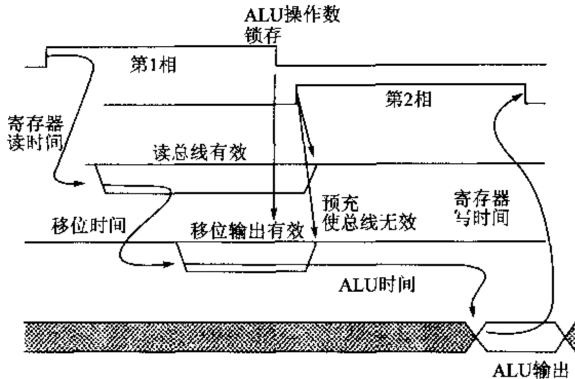
图 4.9 ARM 数据通路的时序(3 级流水线)
