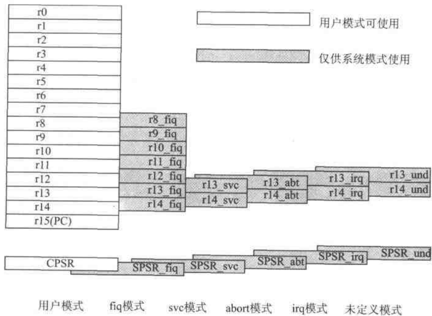
图 2.1 ARM 的可见寄存器
