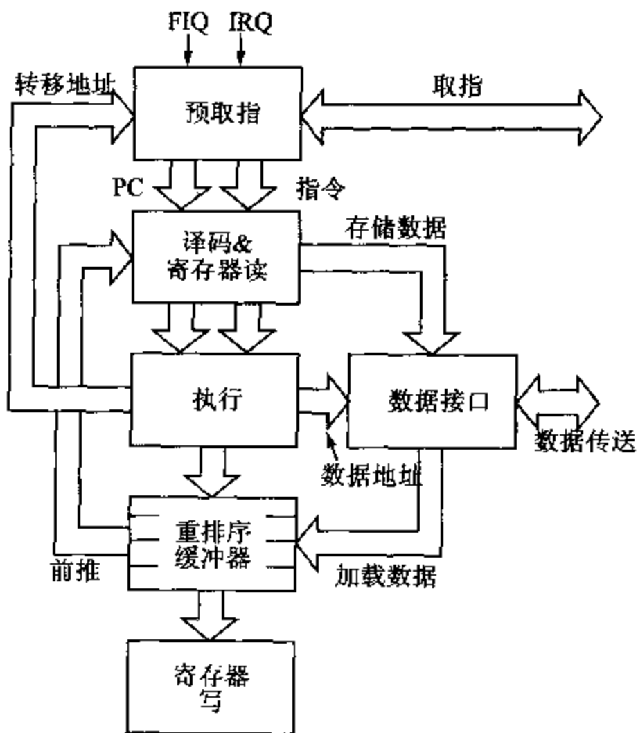
图 14.10 AMULET3 核的组织
