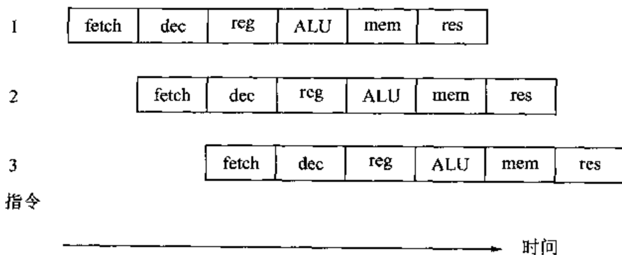
图 1.13 流水线的指令执行
