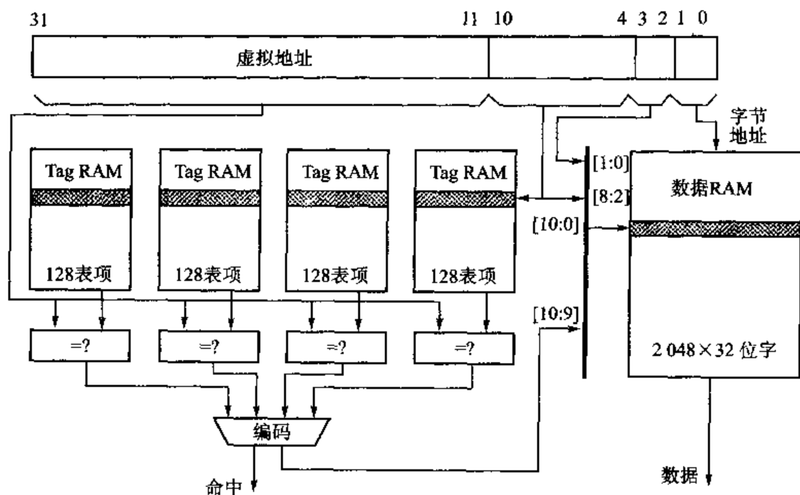
图 12.2 ARM710T Cache 的组织
