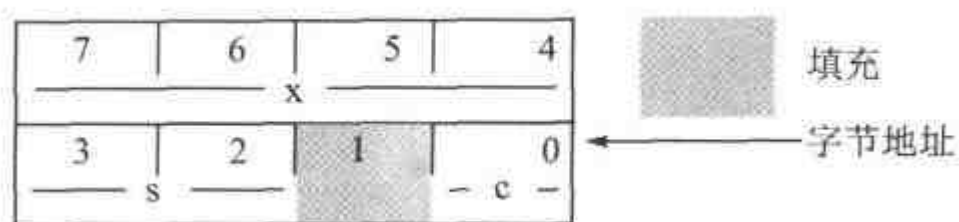
图 6.16 更有效的结构体存储器分配的例子
