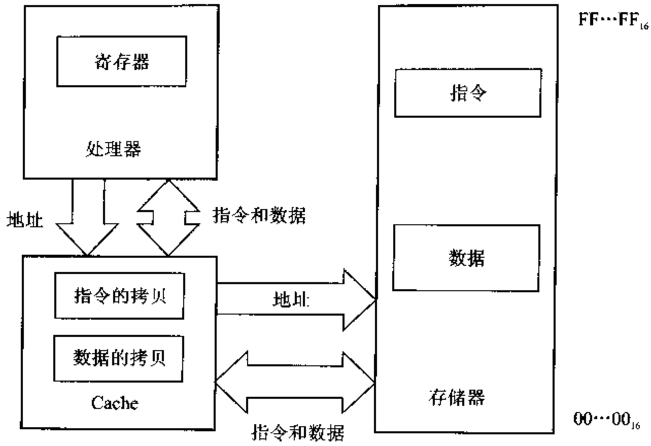
图 10.1 统一的指令和数据 Cache
