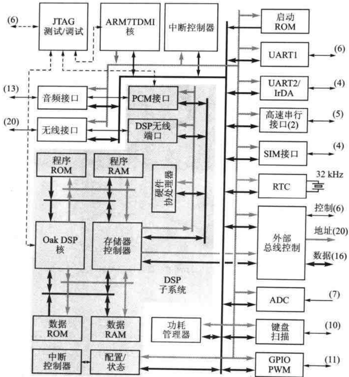
图 13.5 OneC VWS22100 GSM 芯片组织结构
