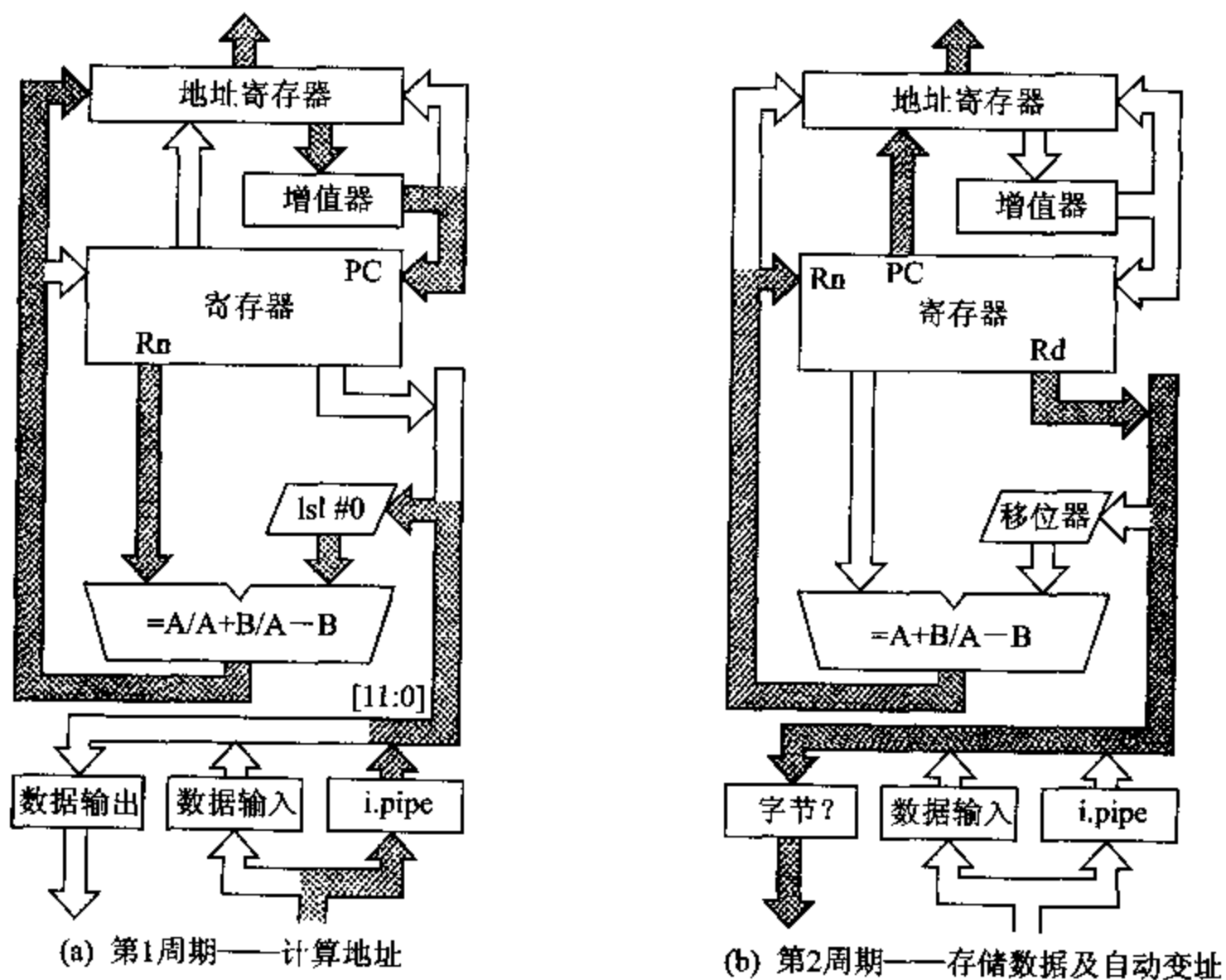
图 4.6 STR(存储寄存器)指令的数据通路行为
