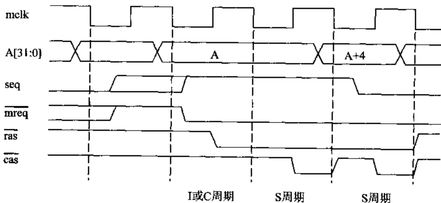
图 8.10 一个内部周期之后的 DRAM 时序
