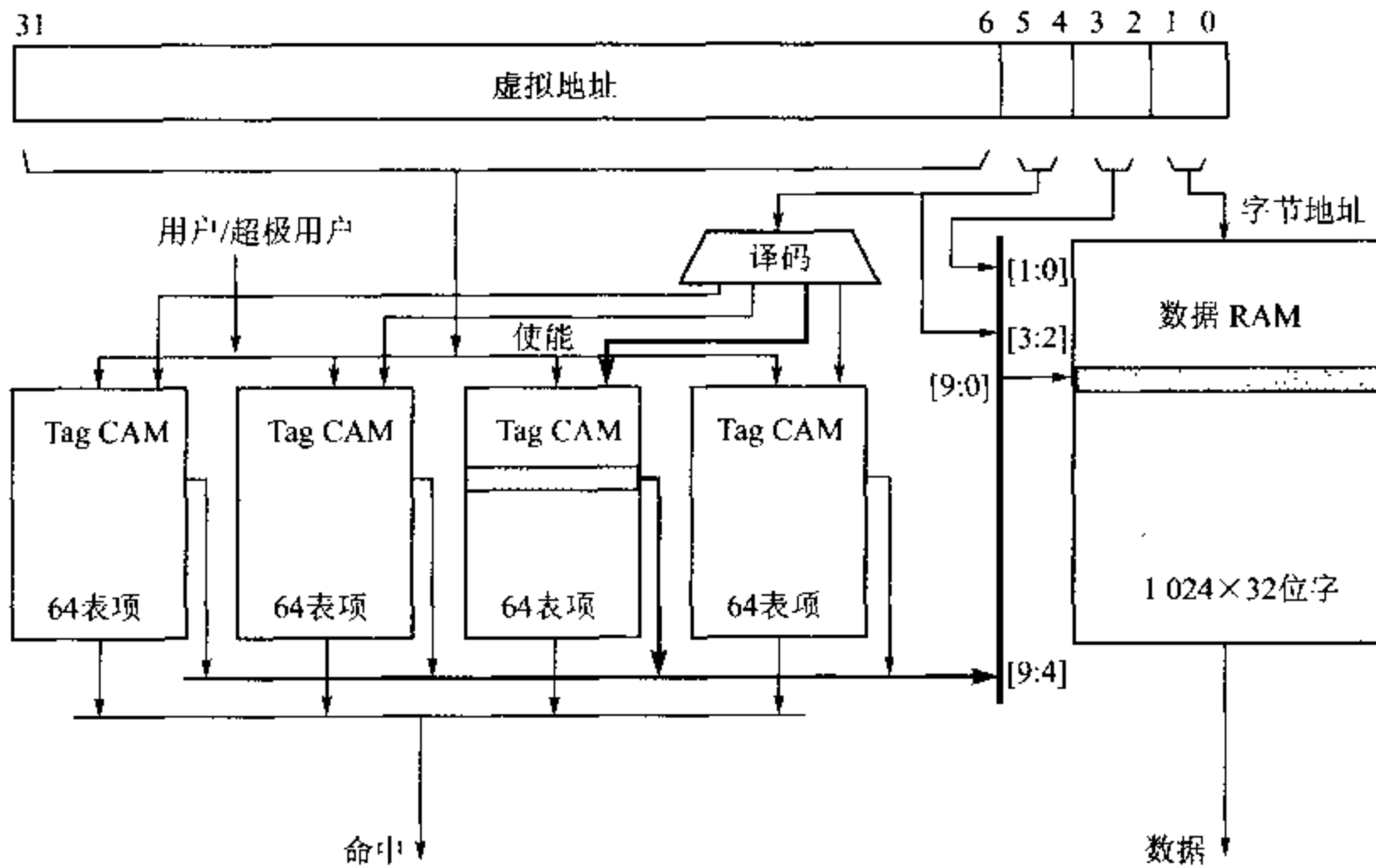
图 10.8 ARM3 的 Cache 组织
