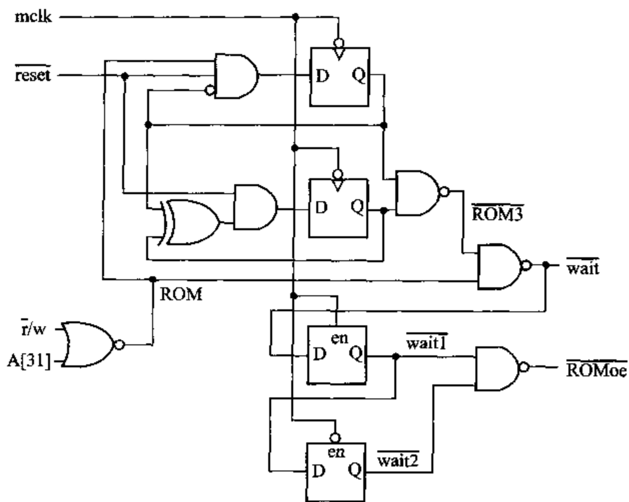
图 8.4 ROM 等待状态产生电路
