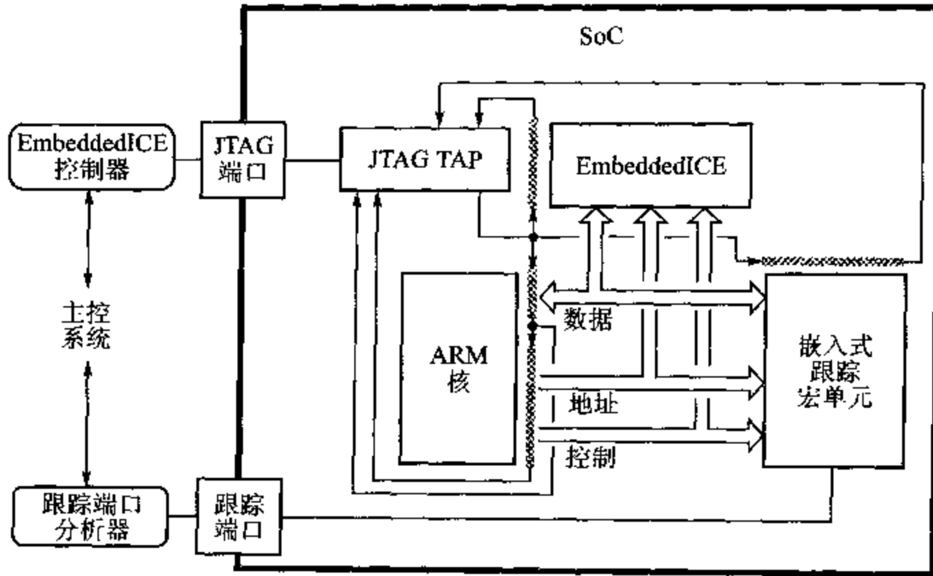
图 8.19 实时调试系统的组织
