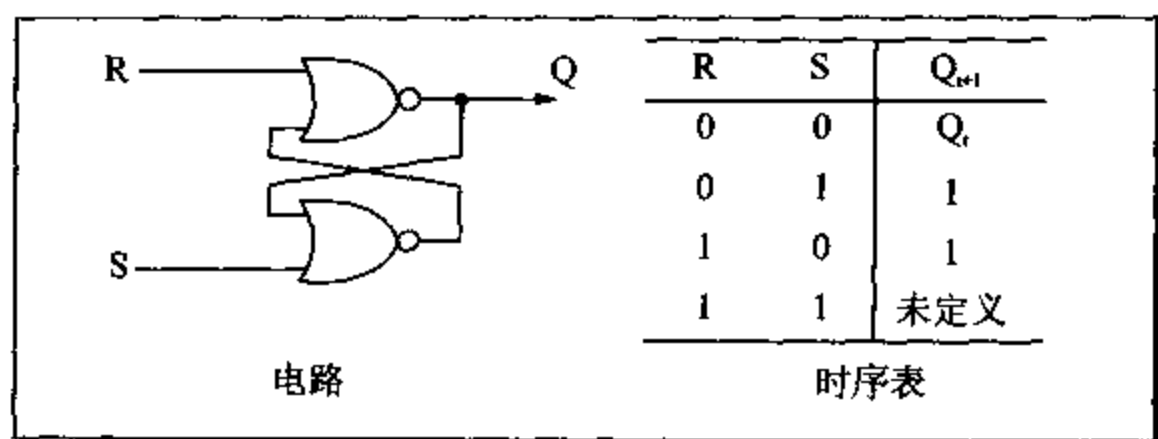
图 A.4 R-S 触发器及其时序表
