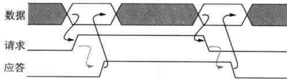
图 14.1 跳变信号通信协议
