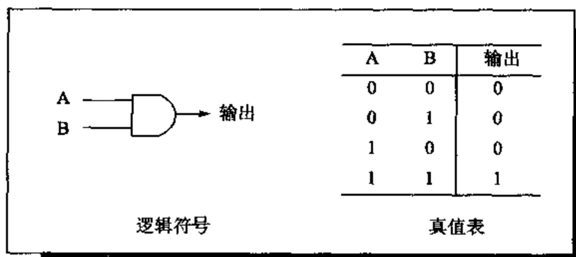
图 A.1 “与”门的逻辑符号和真值表
