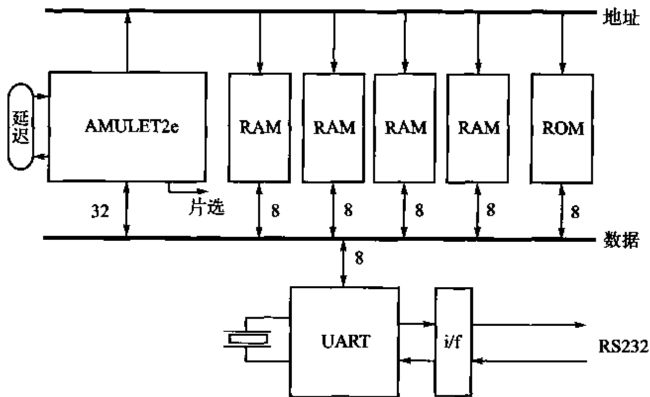
图 14.9 AMULET2e 测试卡的组织
