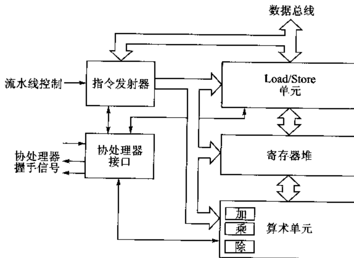
图 6.11 FPA10 的内部组织
