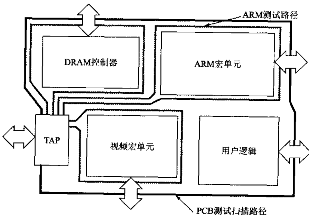
图 8.16 用于宏单元测试的可能的 JTAG 扩展
