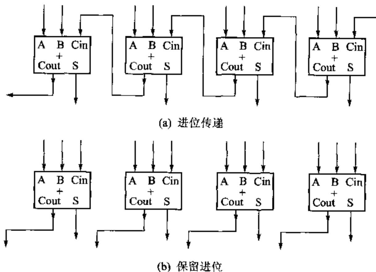
图 4.16 进位传递和保留进位加法器结构
