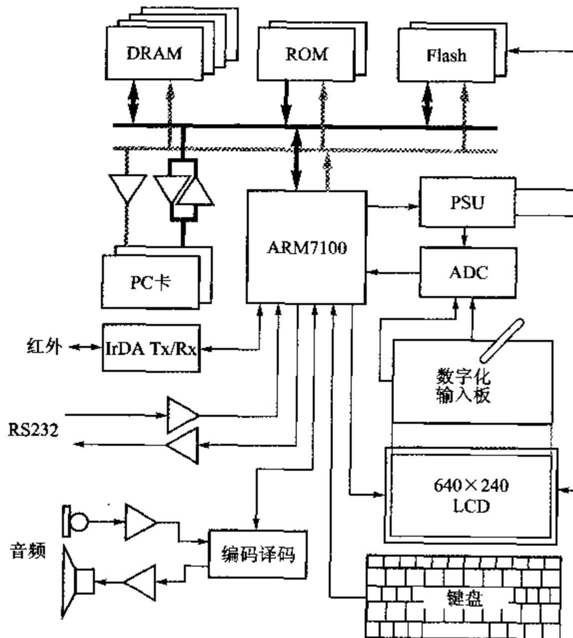
图 13.14 Psion 5 系列的硬件组织
