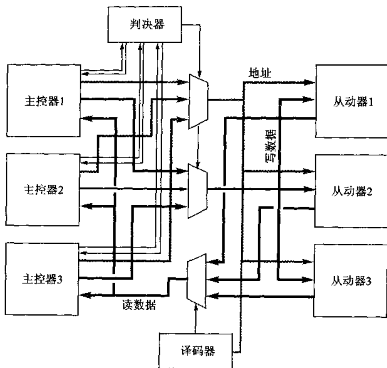
图 8.12 AHB 多路器总线方案
