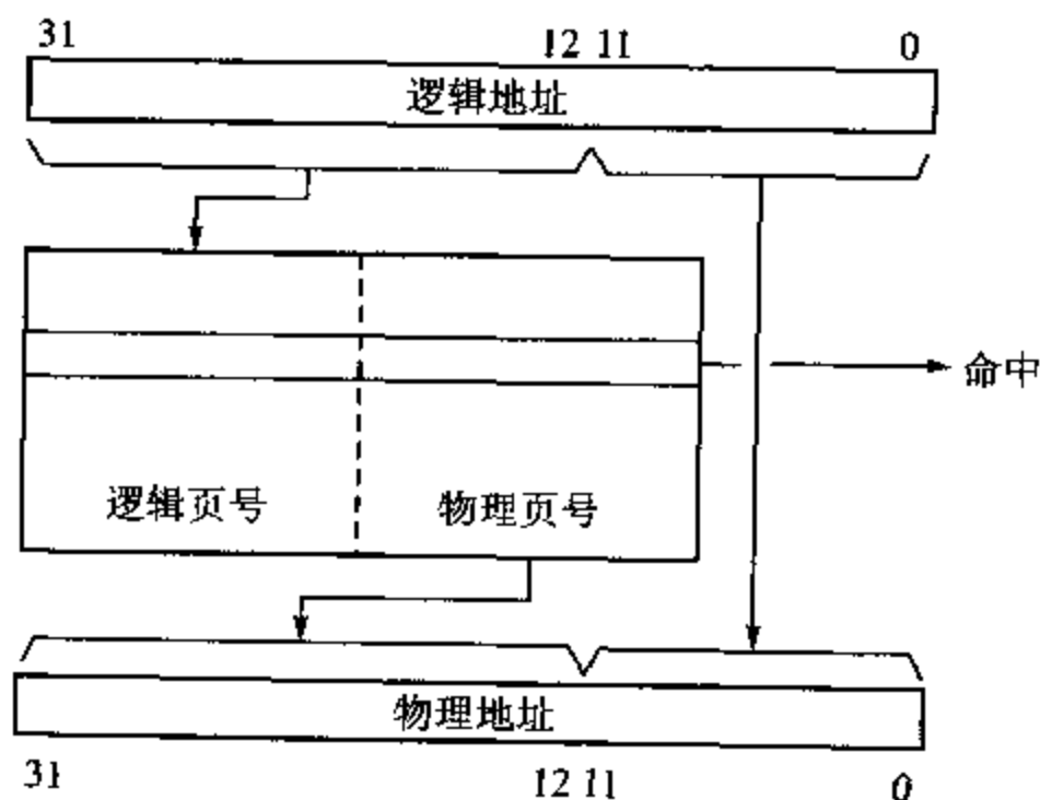
图 10.12 一个 TLB 操作
