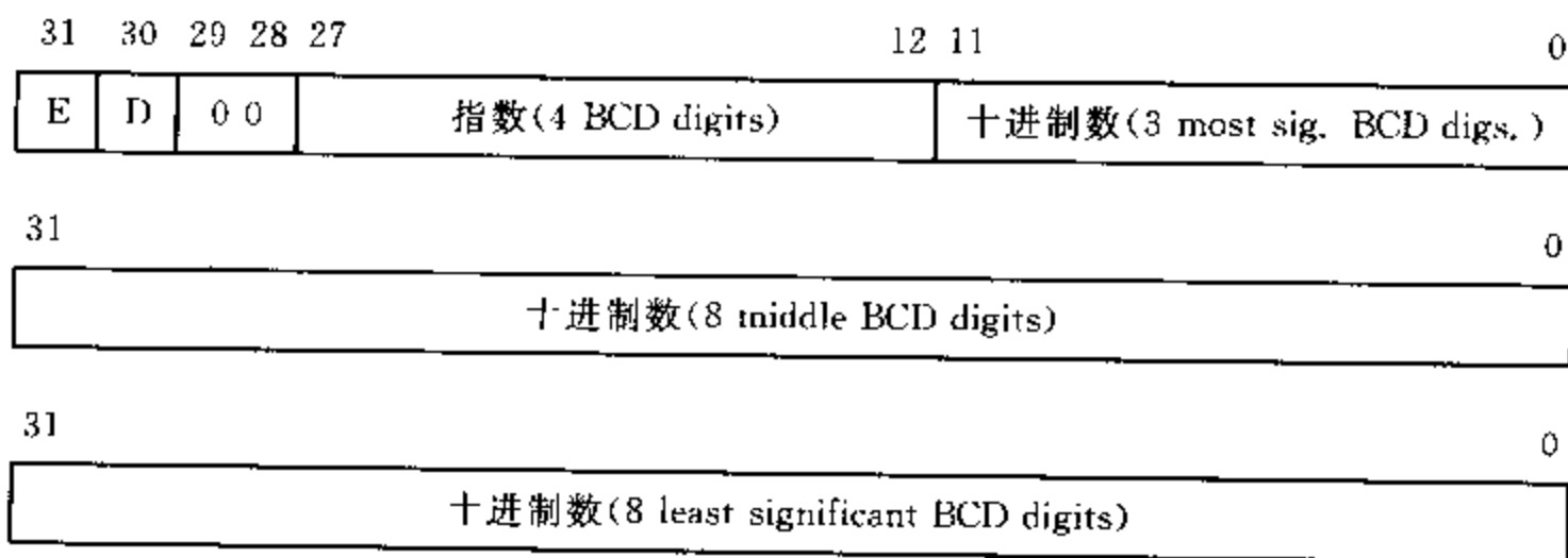
图 6.5 IEEE 754 压缩的十进制浮点数格式
