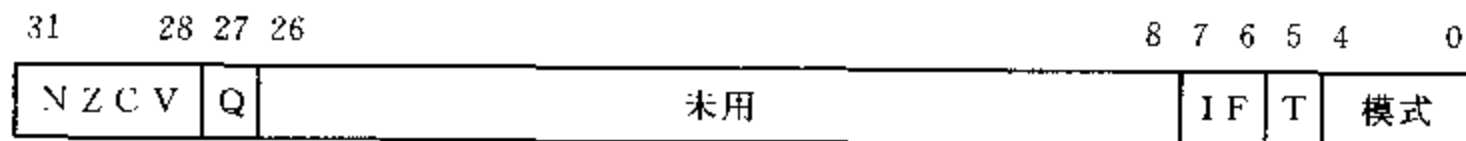
图 8.21 ARM v5TE PSR 格式
