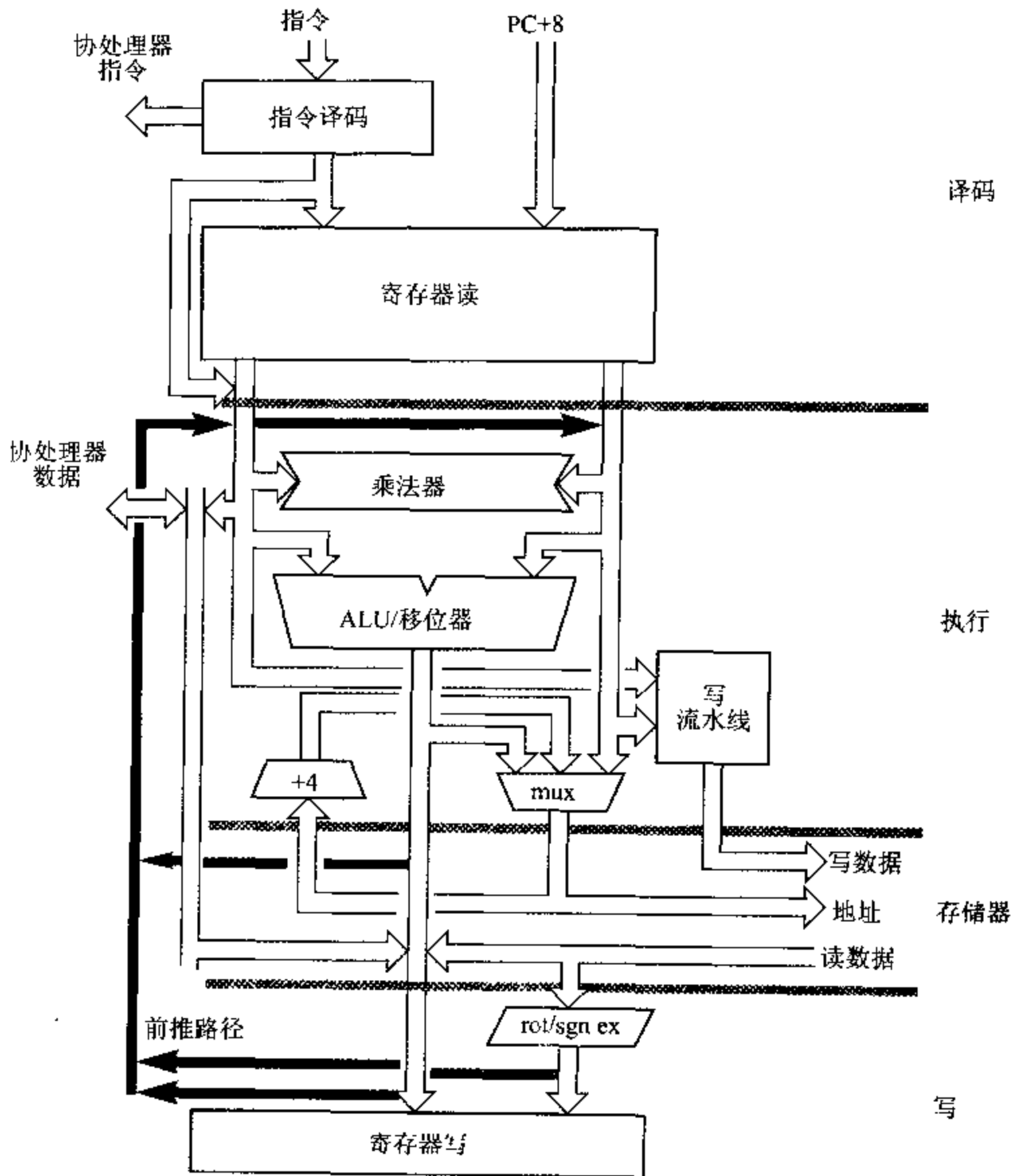
图 9.6 ARM8 整数单元的组织
