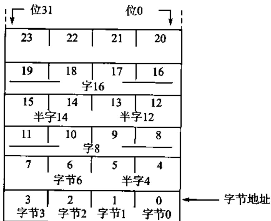
图 2.3 ARM 的存储器组织
