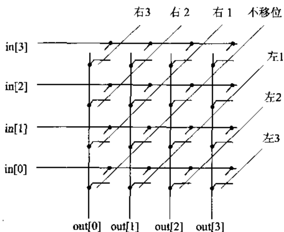
图 4.15 交叉开关桶式移位器原理
