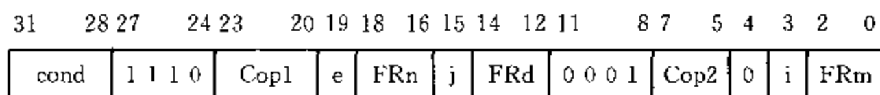
图 6.9 浮点数据操作的二进制编码
