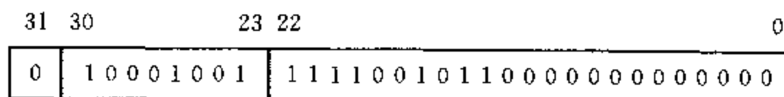
图 6.2 1995 的 IEEE 754 单精度表示
