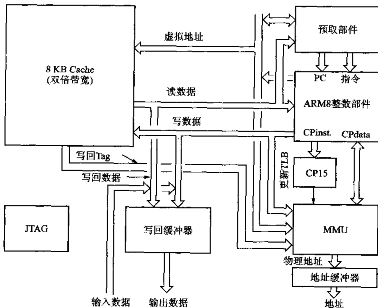
图 12.5 ARM810 的组织
