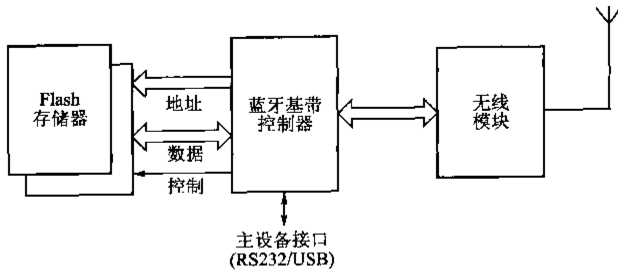
图 13.8 典型的蓝牙应用
