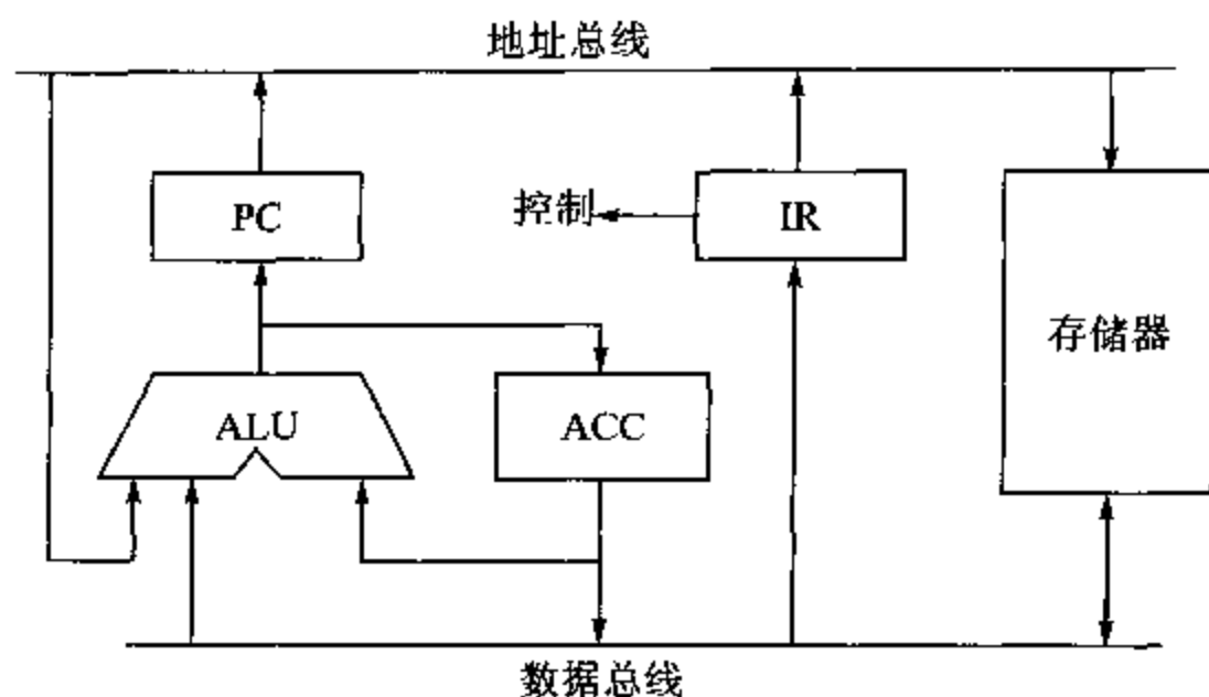
图 1.5 MU0 数据通路示例
