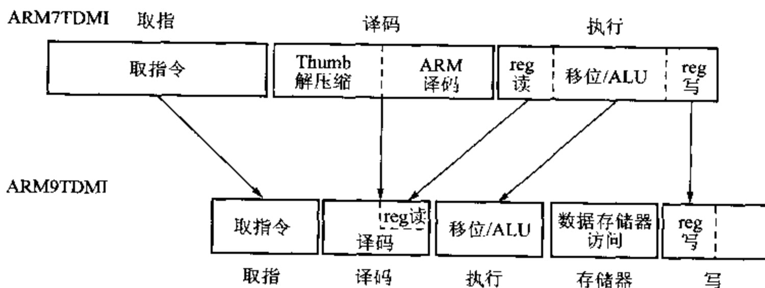
图 9.7 ARM7TDMI 与 ARM9TDMI
