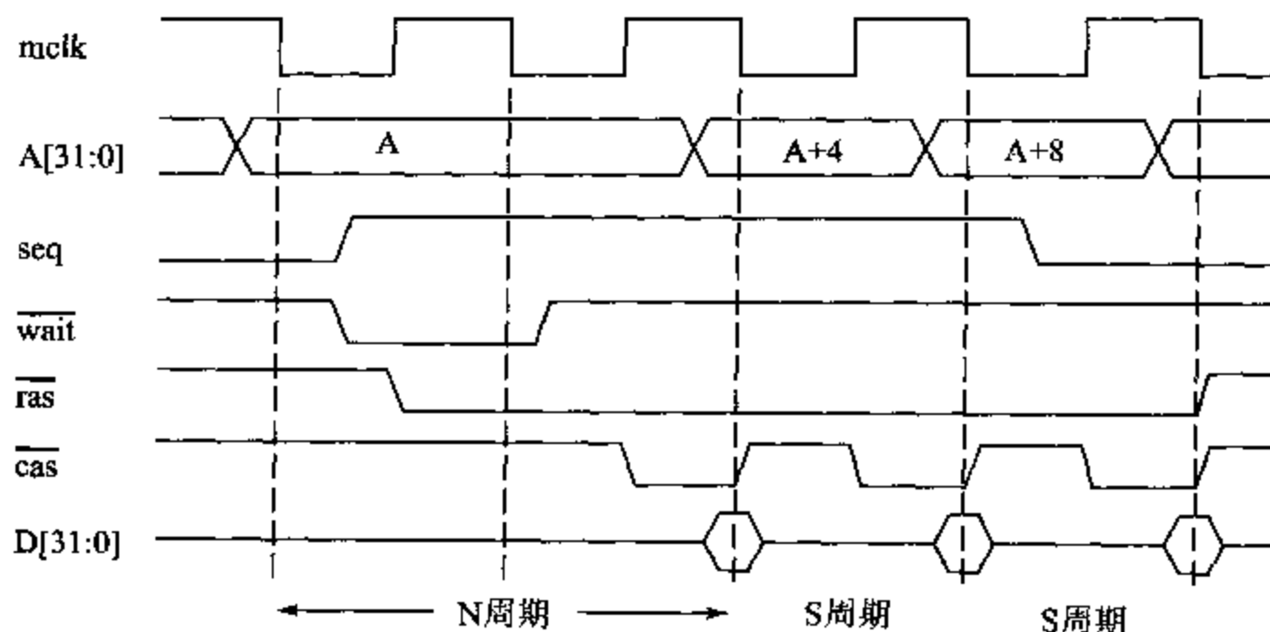
图 8.9 DRAM 时序图
