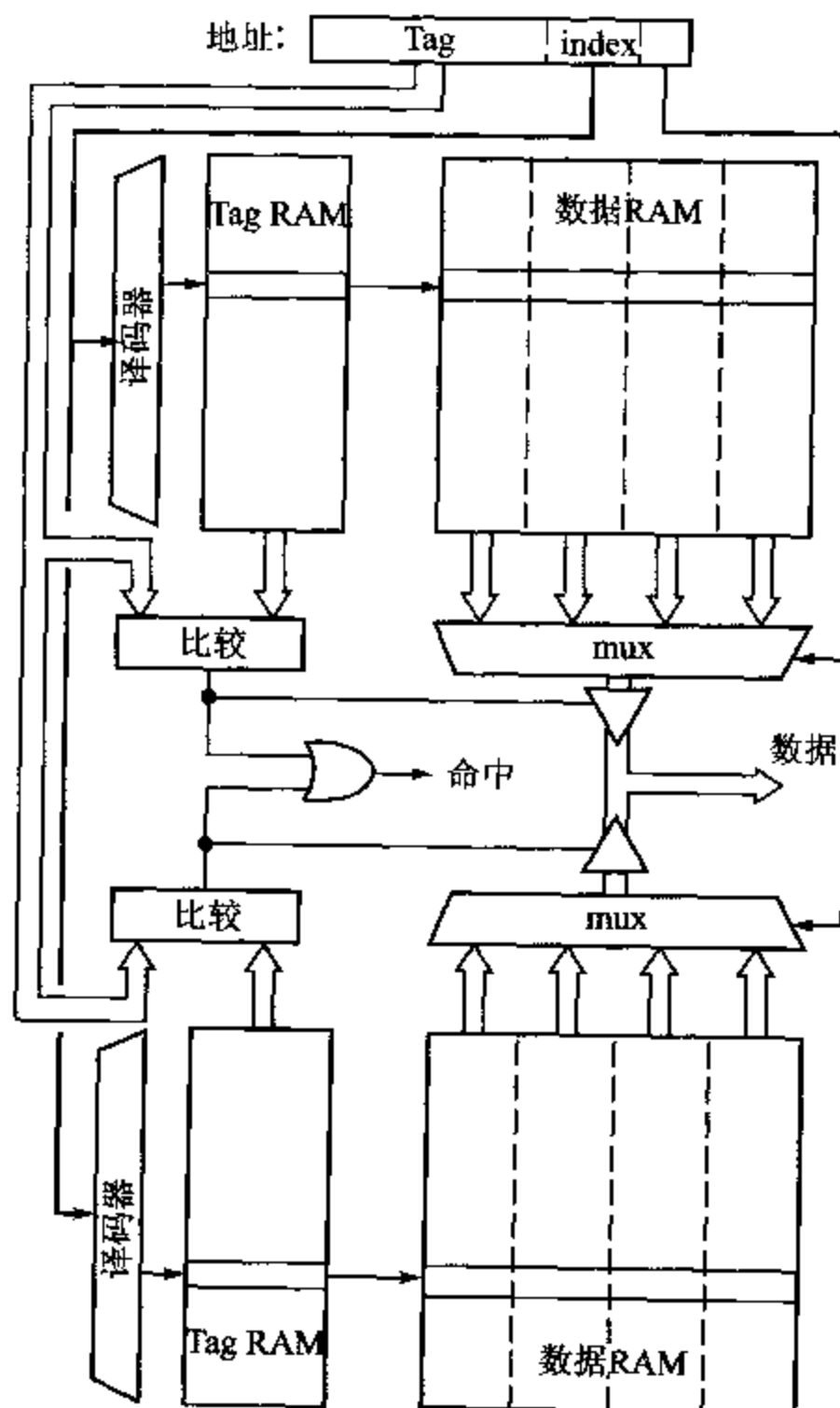
图 10.4 两路组相联 Cache 组织
