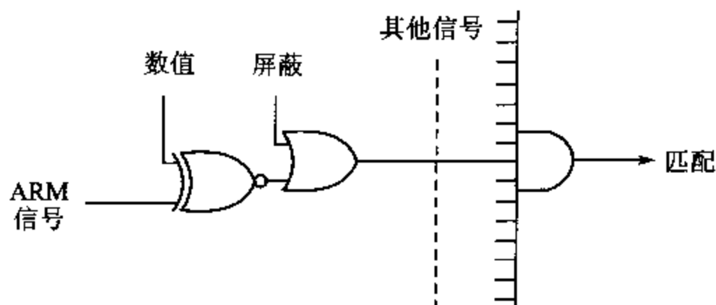
图 8.17 EmbeddedICE 信号比较逻辑
