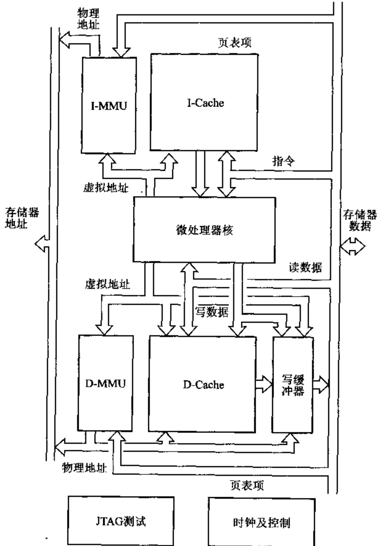
图 12.7 StrongARM 组织
