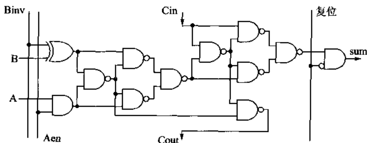
图 1.7 MU0 ALU 逻辑的一位
