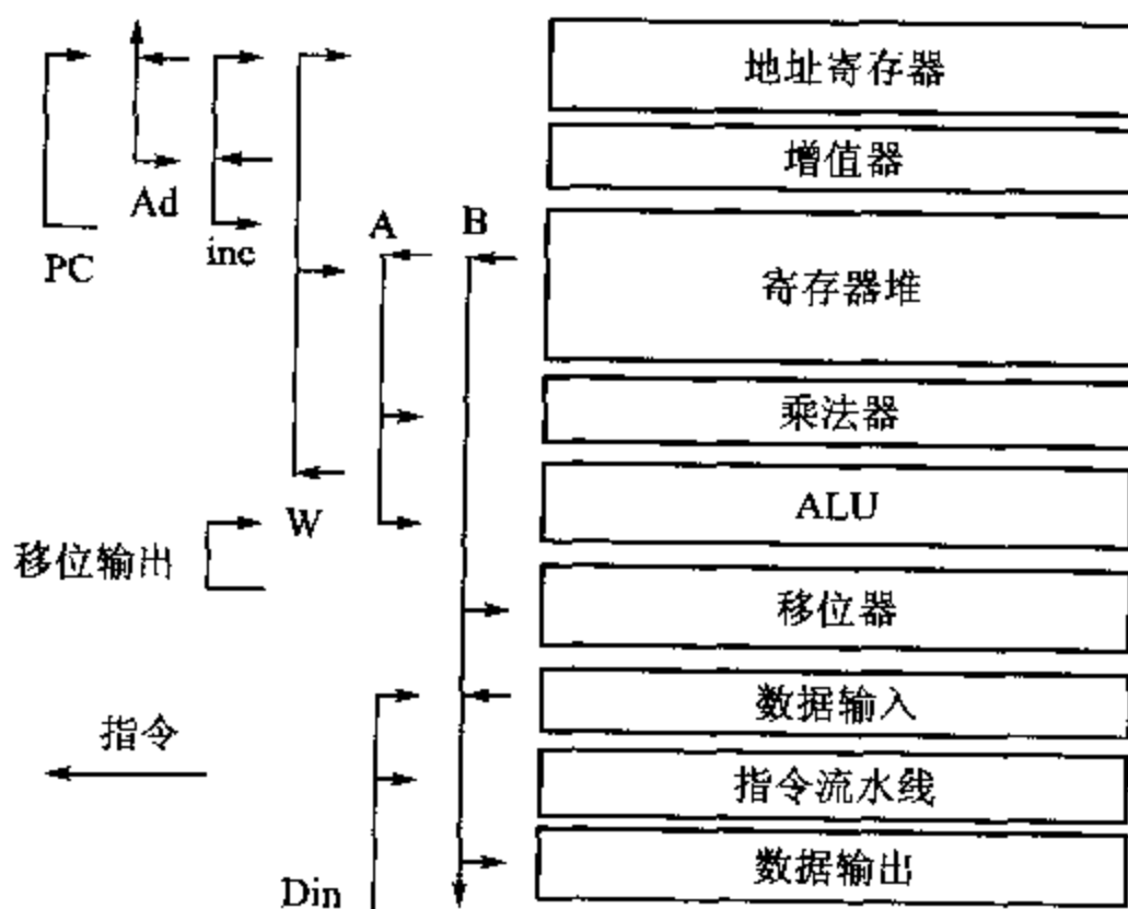
图 4.20 ARM 核的数据通路总线
