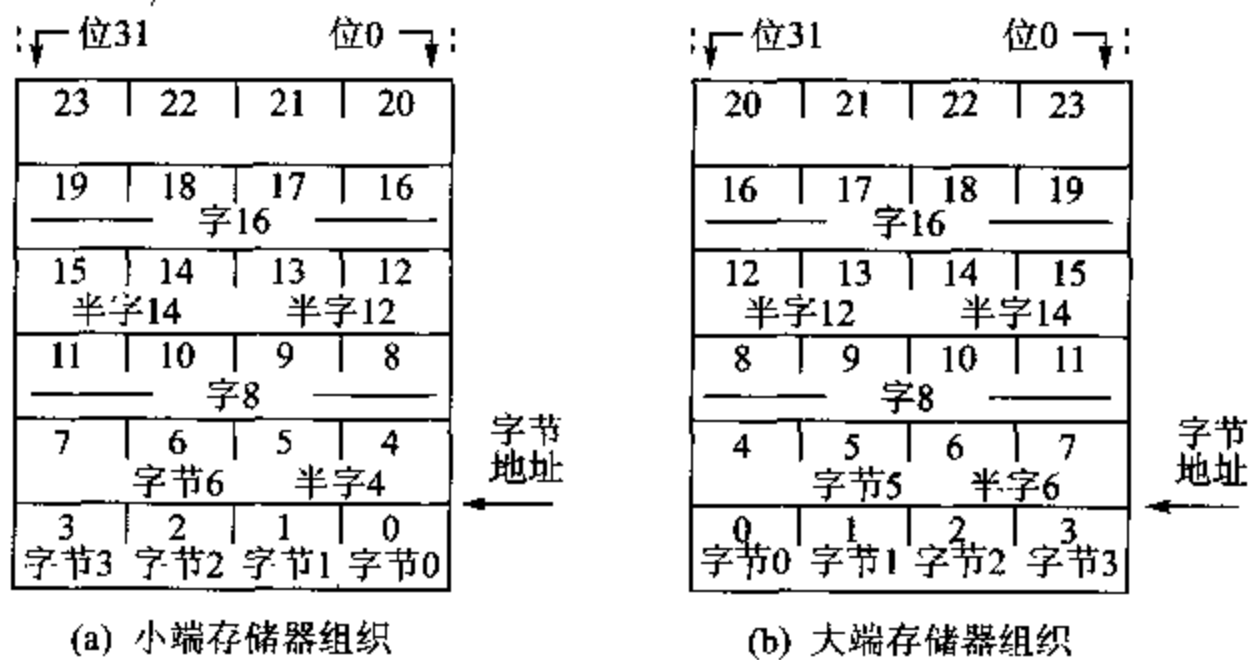
图 5.1 小端和大端存储器组织
