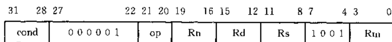
图 5.19 算术指令扩展空间
