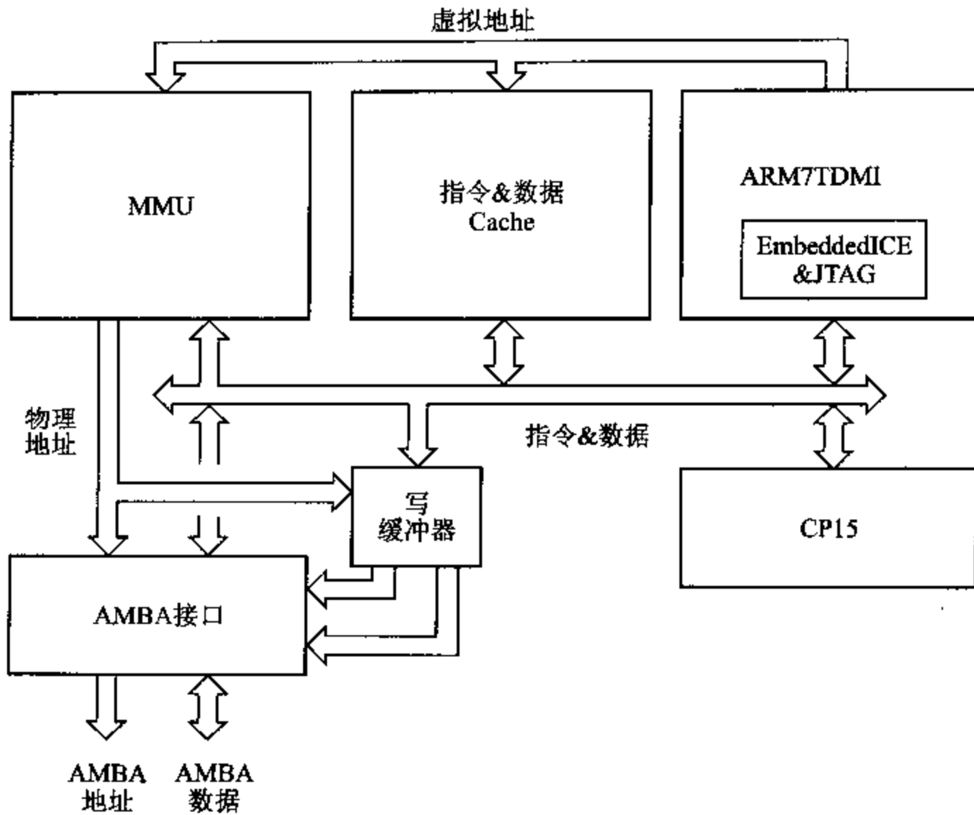
图 12.1 ARM710T 和 ARM720T 的组织结构
