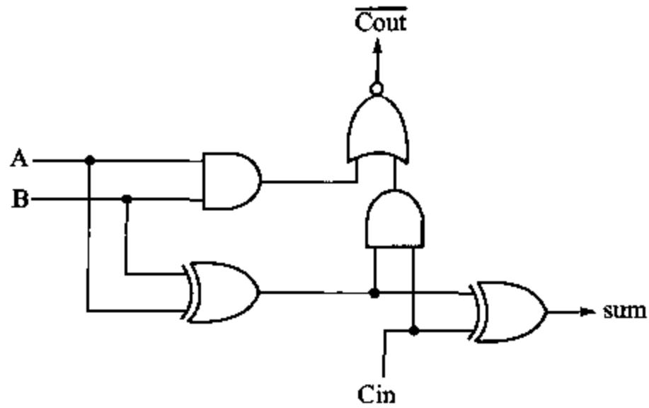
图 4.10 原用于 ARM1 的行波进位加法器电路
