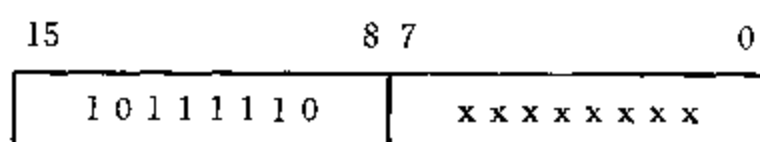
图 7.7 Thumb 断点指令二进制编码
