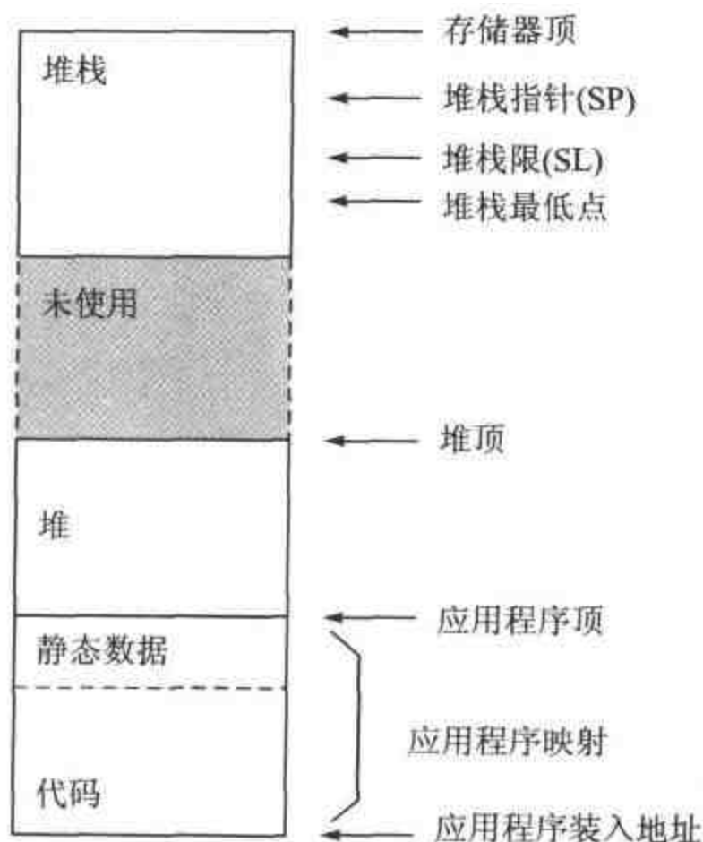
图 6.13 标准的 ARM C 程序地址空间模型
