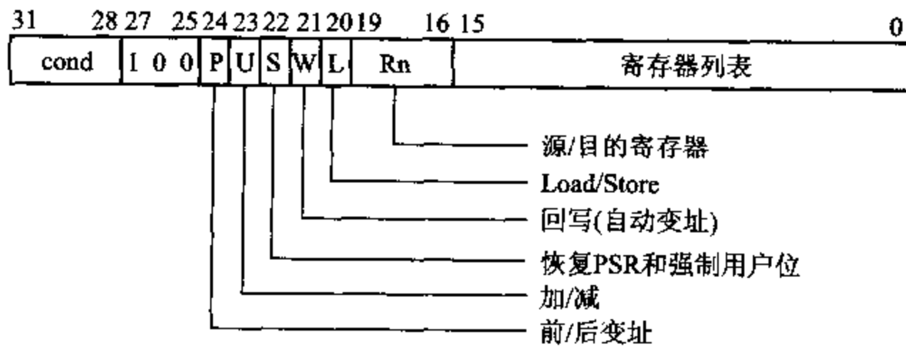
图 5.11 多寄存器数据传送指令的二进制编码
