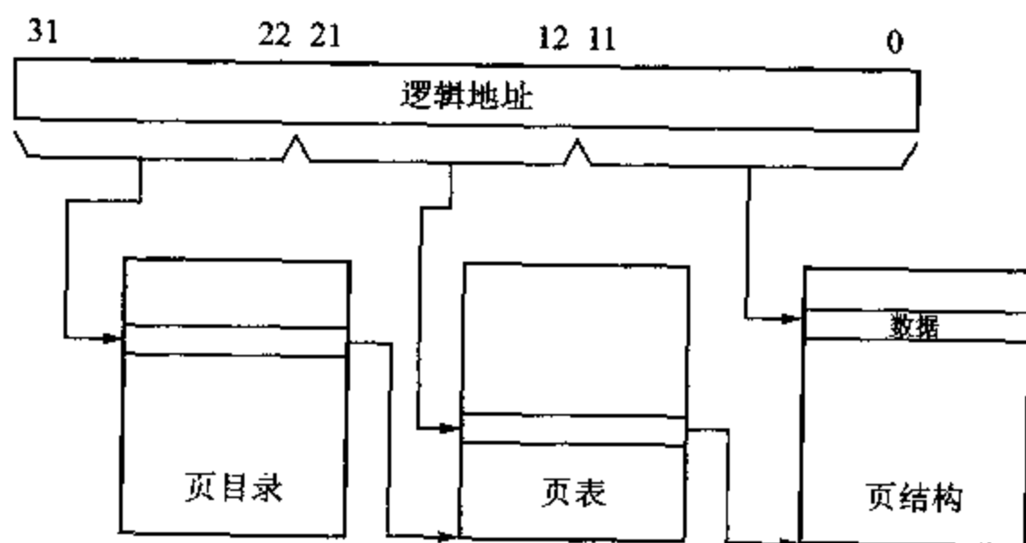
图 10.11 页式存储器管理方案
