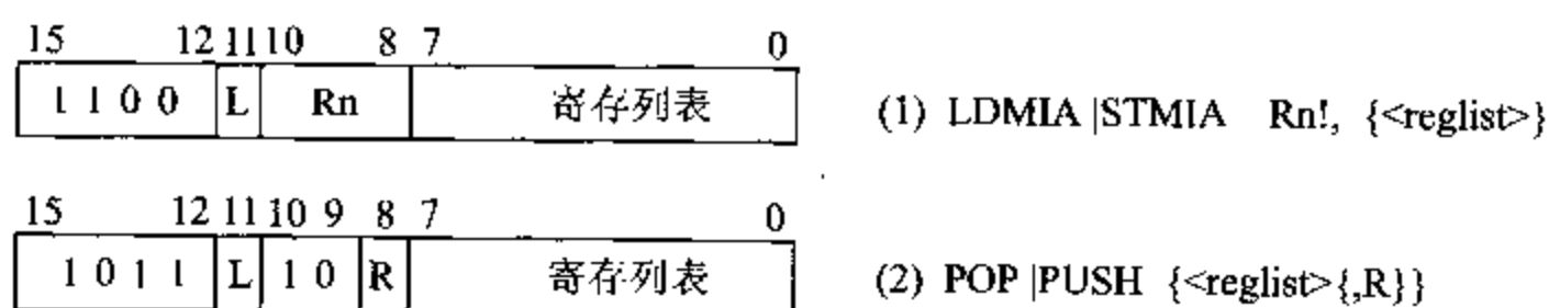
图 7.6 Thumb 多寄存器传送指令的二进制编码
