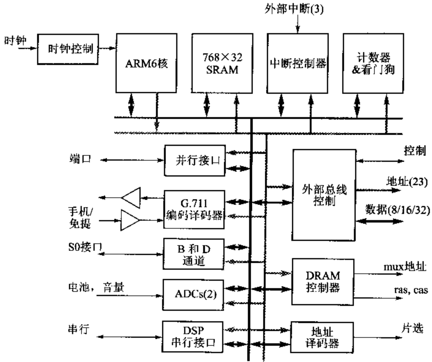
图 13.2 VIP 的组织结构
