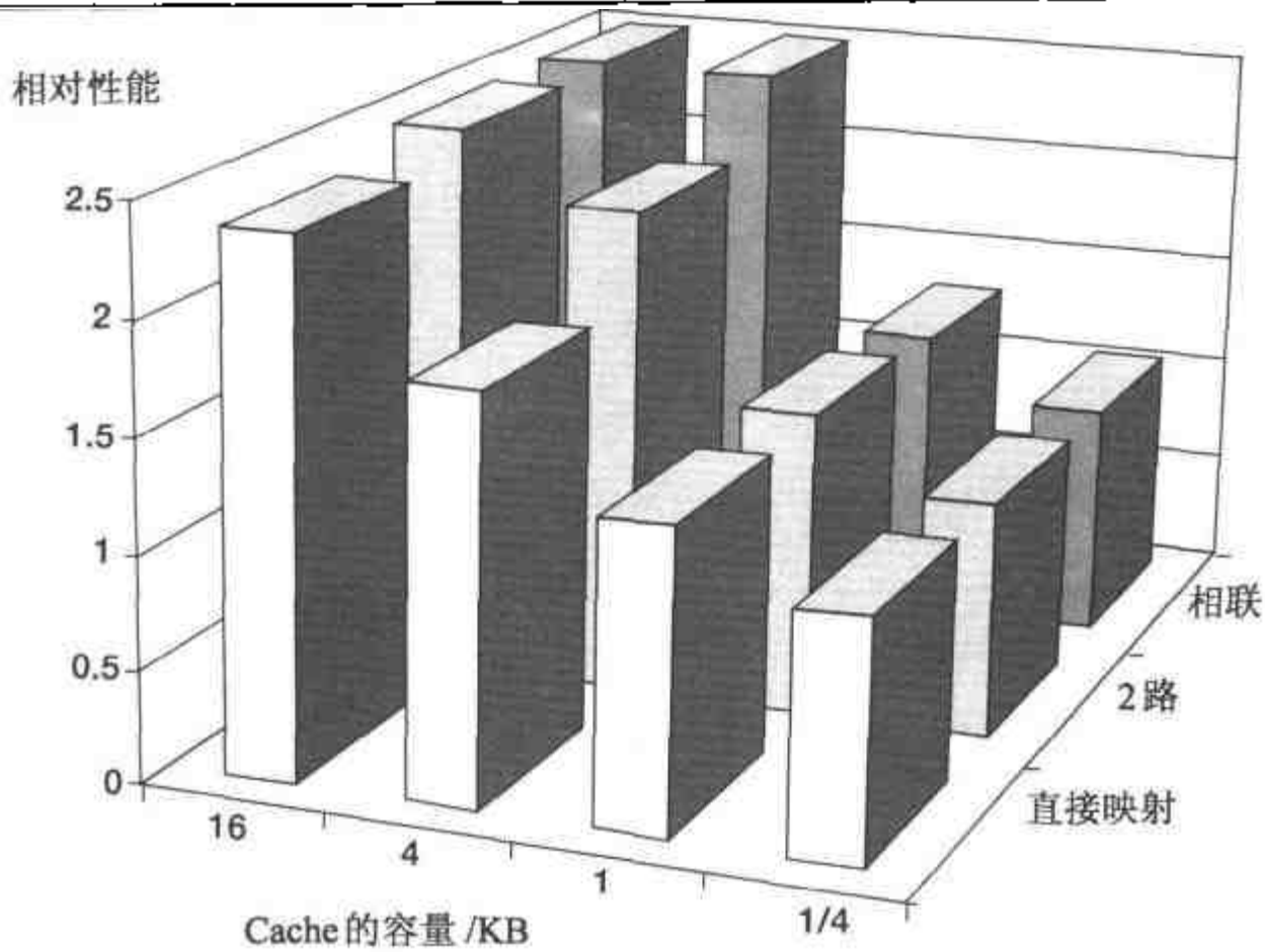
图 10.6 以容量和组织为函数的统一 Cache 性能
