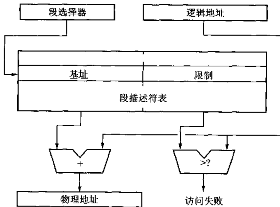
图 10.10 段式存储器管理方法
