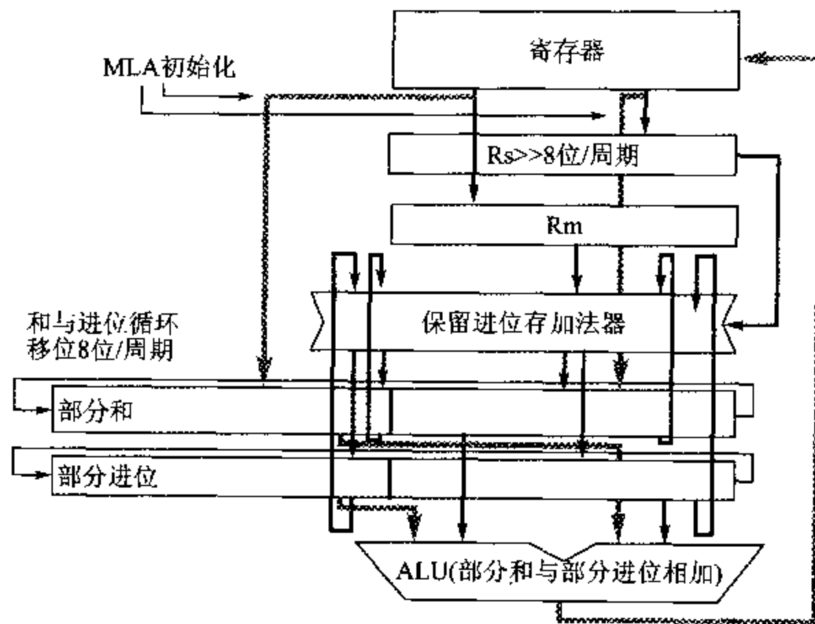
图 4.17 ARM 高速乘法器组织结构
