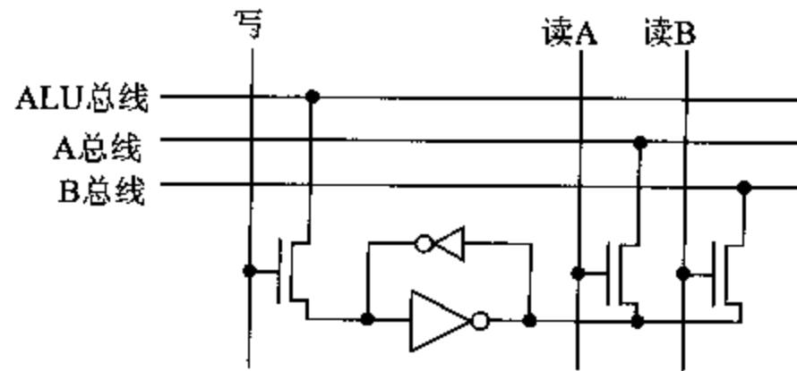
图 4.18 ARM6 的寄存器单元电路
