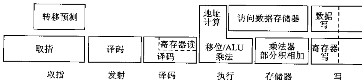
图 9.9 ARM10TDMI 的流水线
