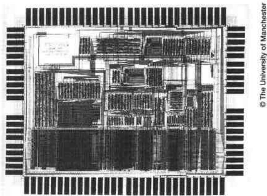
图 14.5 AMULET1 版图
