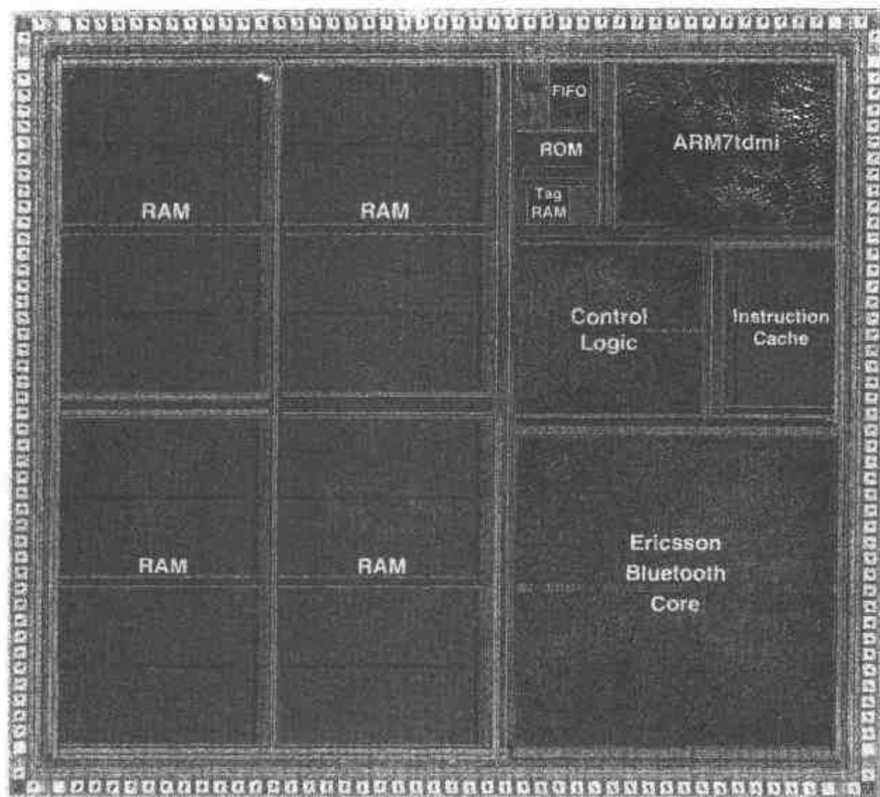
图 13.9 蓝牙基带控制器管芯照片
