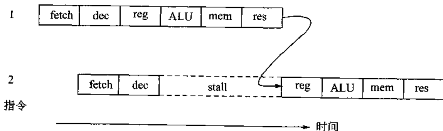
图 1.14 先写后读的流水线冒险
