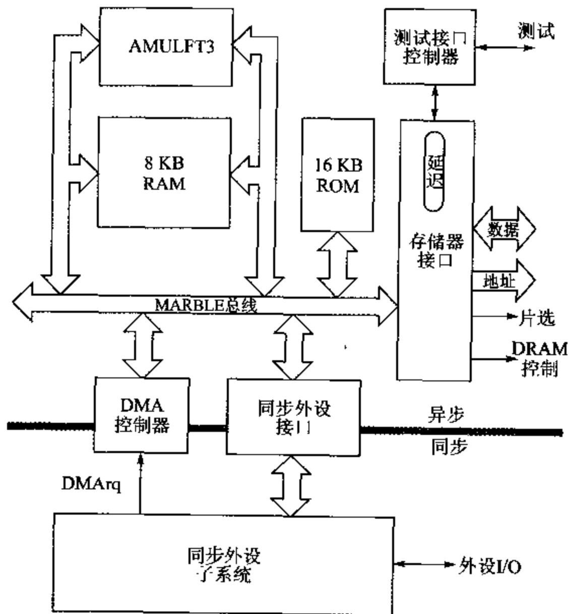
图 14.12 AMULET3H 的异步子系统
