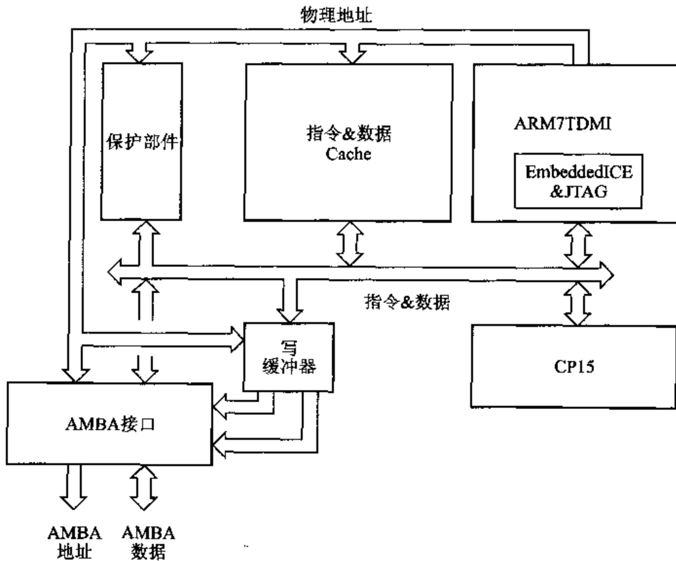
图 12.4 ARM740T 组织
