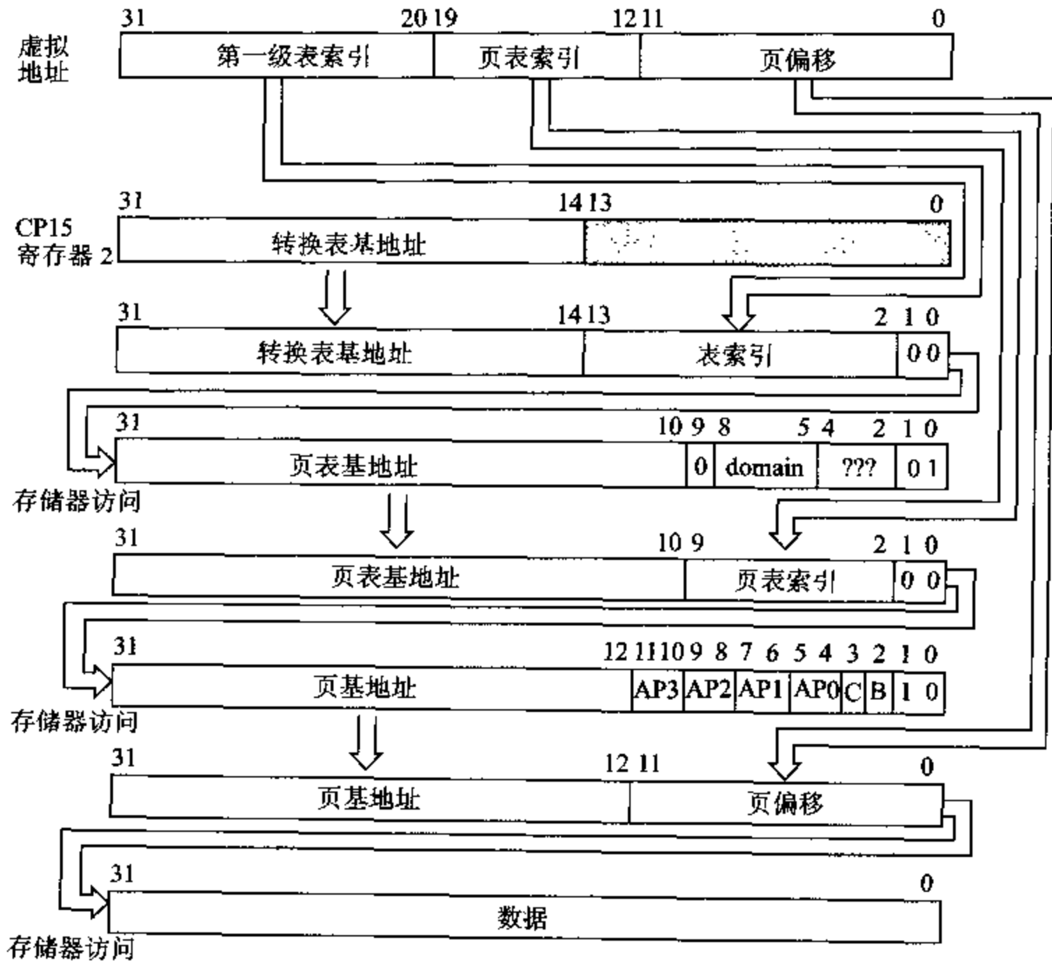
图 11.5 小页转换次序
