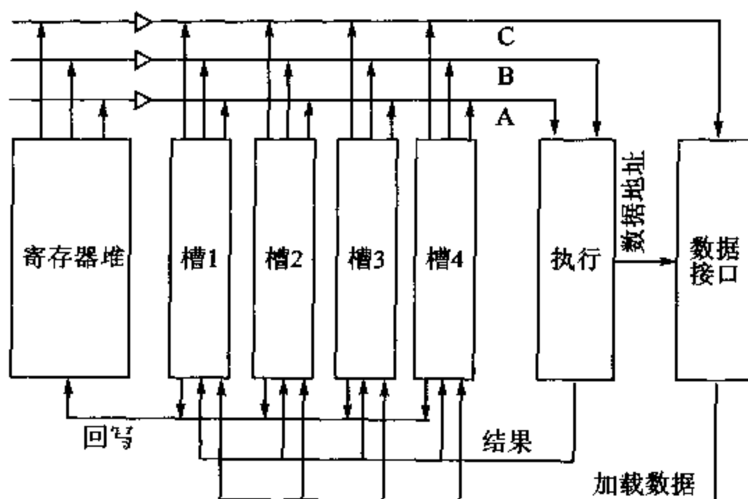
图 14.11 AMULET3 重排序缓冲器的组织
