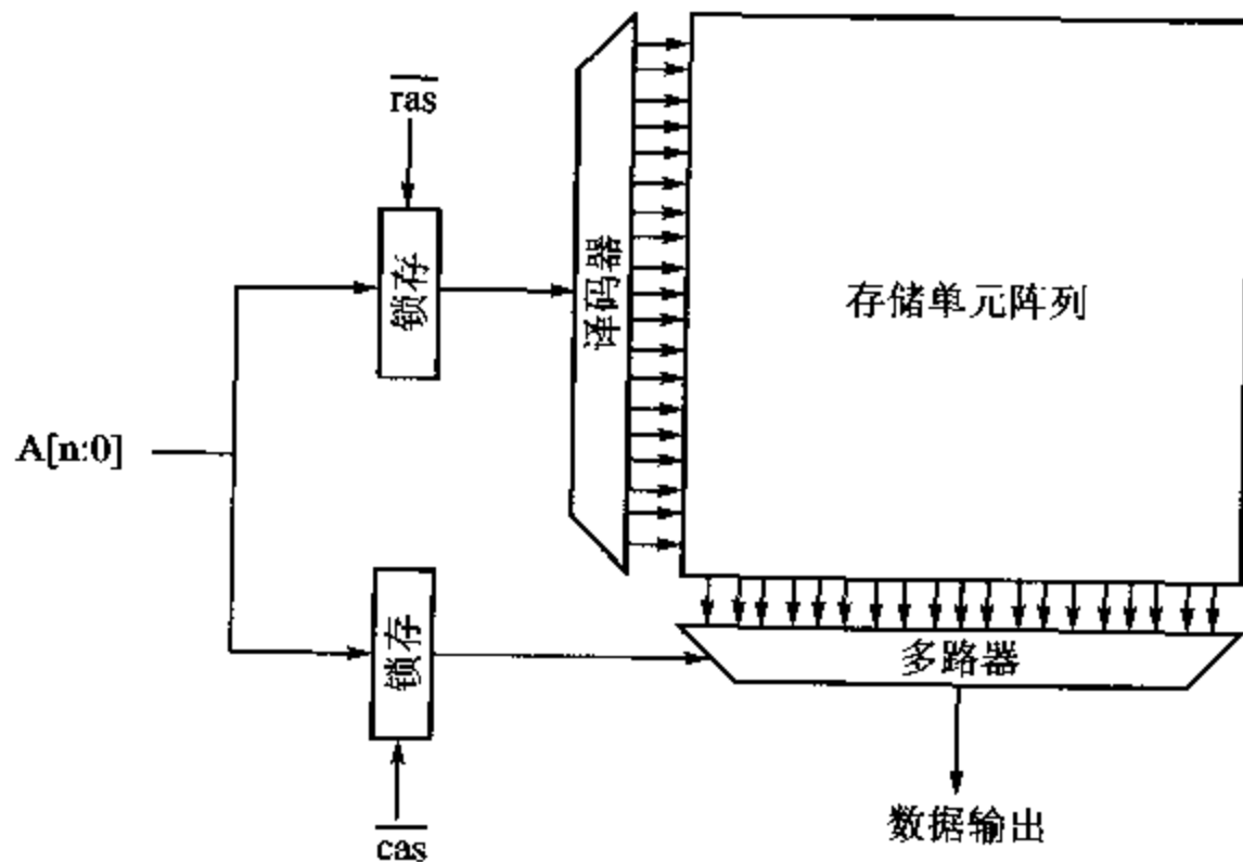
图 8.7 DRAM 存储器的组织
