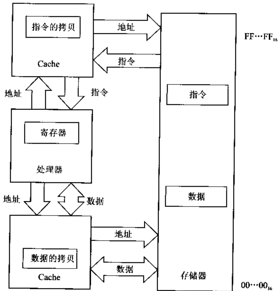
图 10.2 数据和指令分开的 Cache
