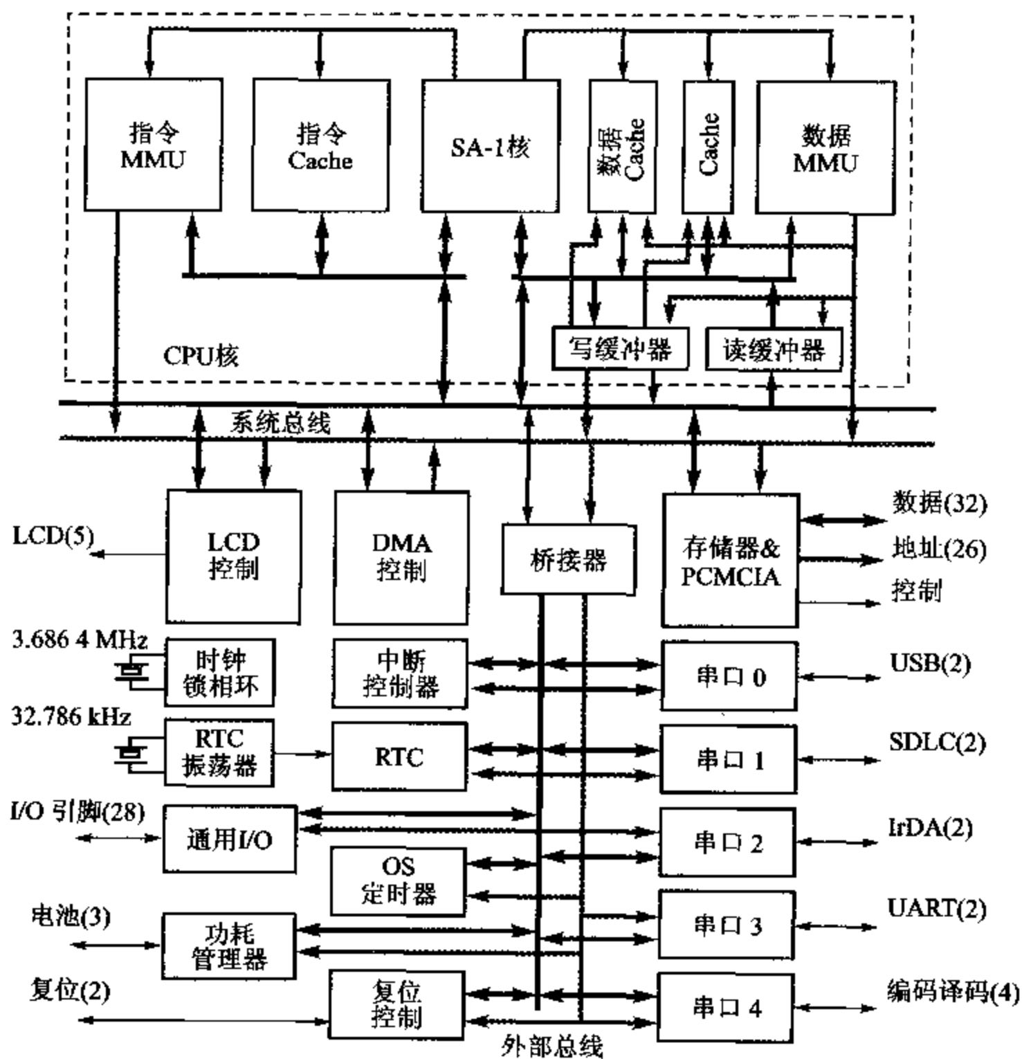
图 13.16 SA-1100 组织结构
