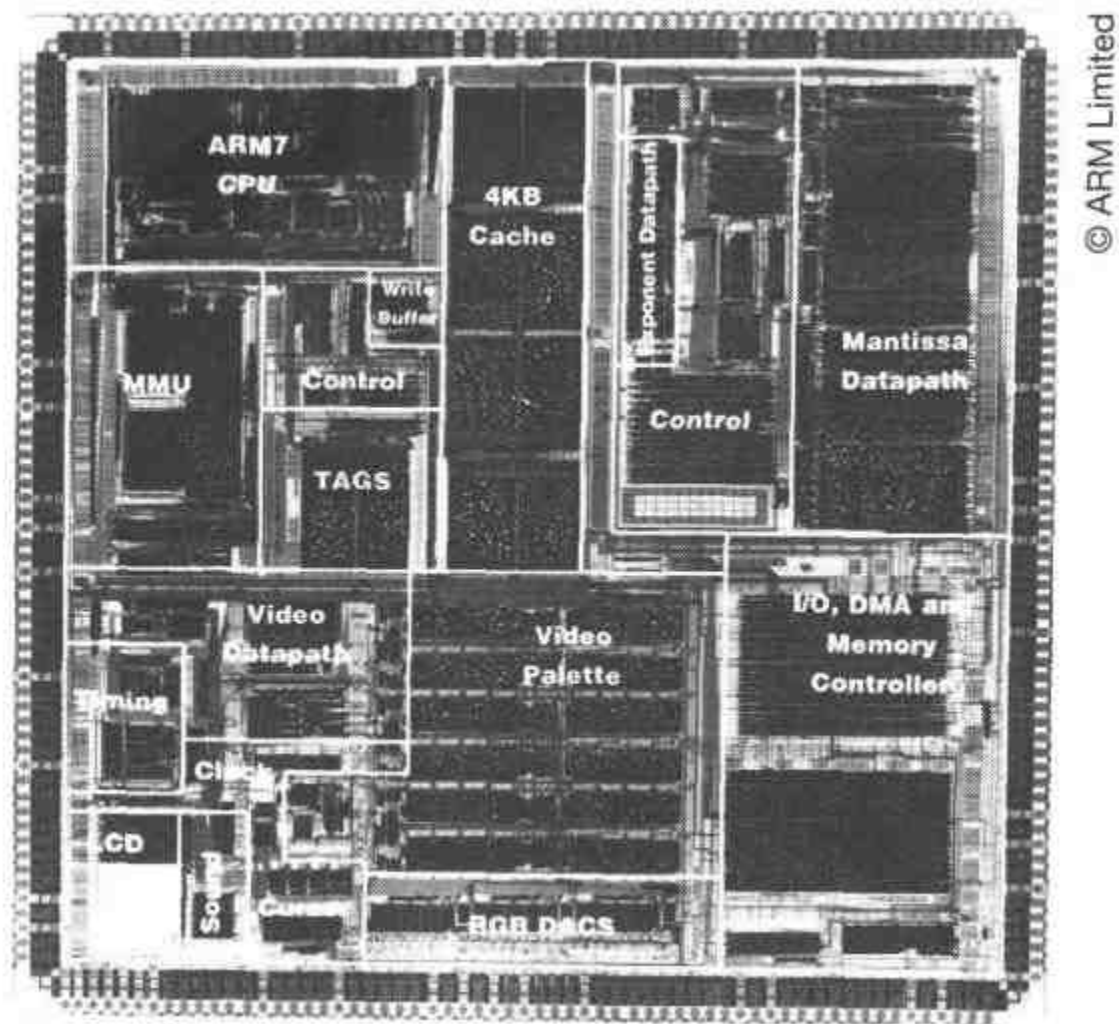
图 13.11 ARM7500FE 的管芯照片
