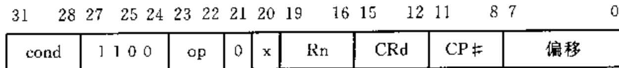
图 5.22 协处理器指令扩展空间
