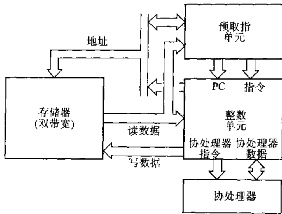
图 9.5 ARM8 处理器核的组织
