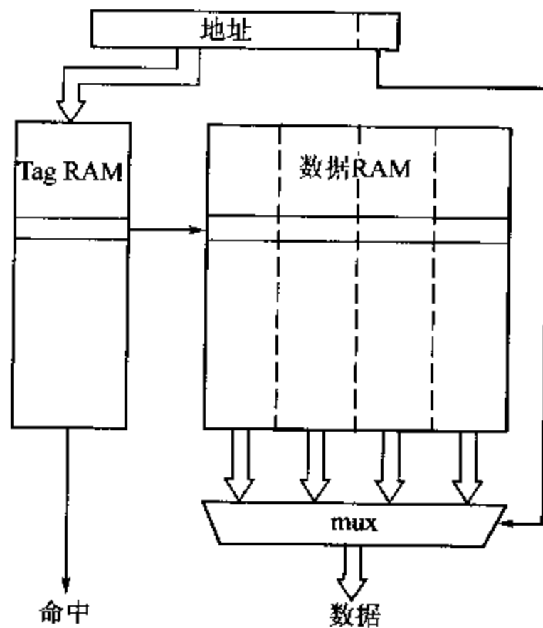
图 10.5 全相联 Cache 组织
