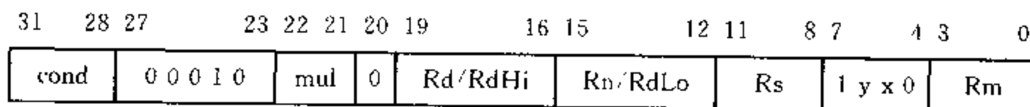
图 8.22 v5TE 体系结构乘法指令的二进制编码
