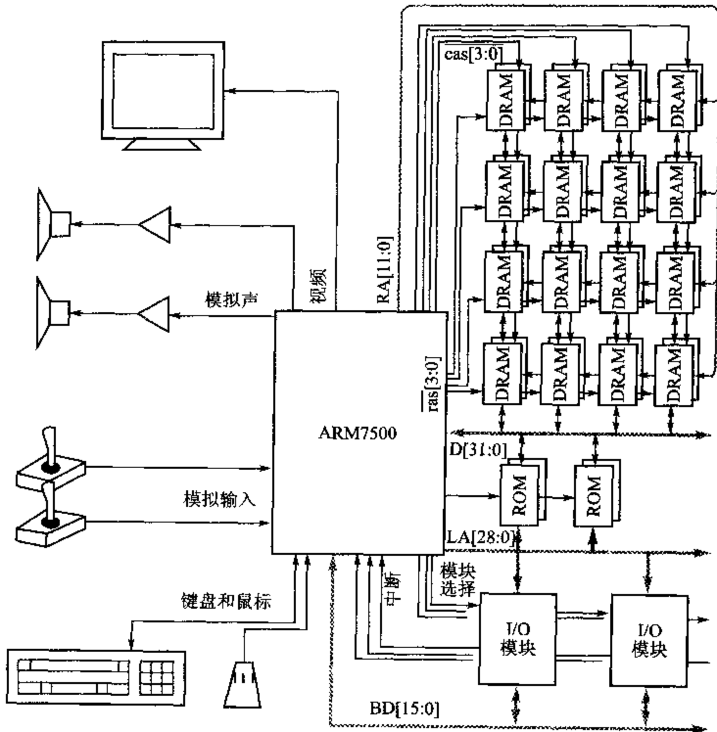
图 13.10 典型的 ARM7500 系统组织结构
