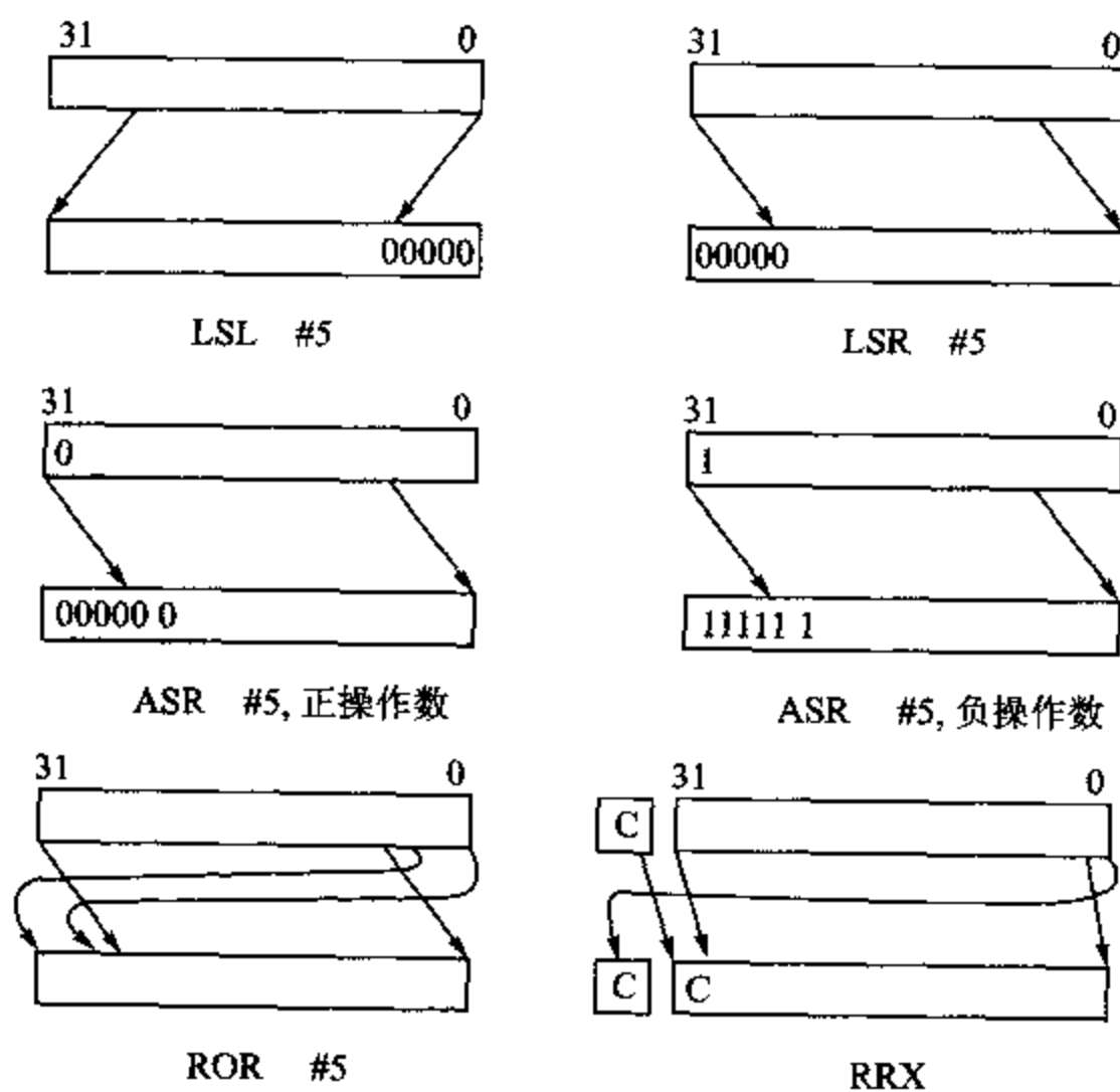
图 3.1 ARM 移位操作
