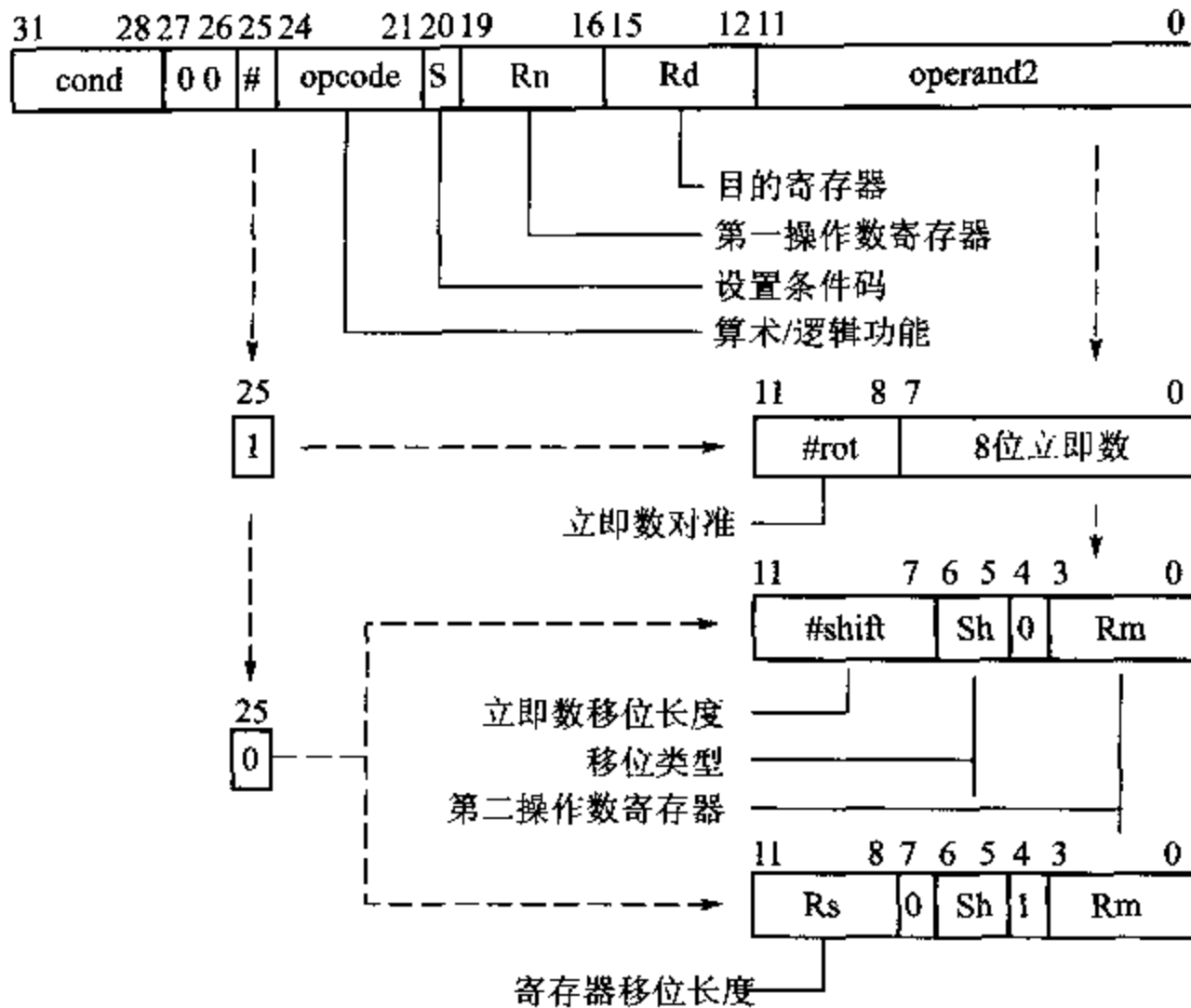
图 5.6 数据处理指令的二进制编码
