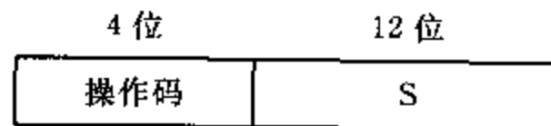
图 1.4 MU0 的指令格式
