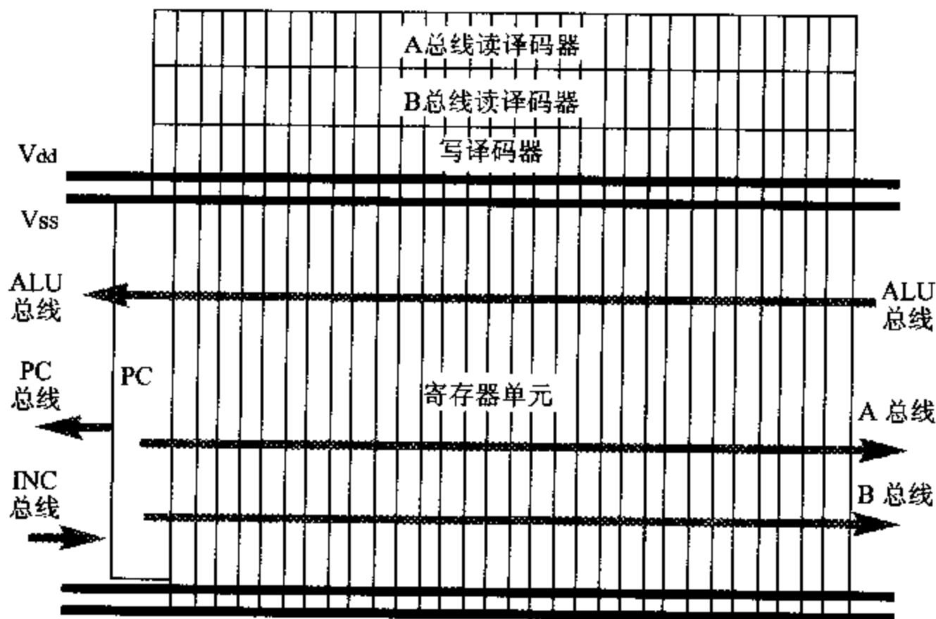
图 4.19 ARM 寄存器堆的版图规划
