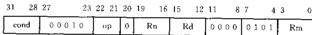
图 8.23 v5TE 体系结构加法/减法指令的二进制编码
