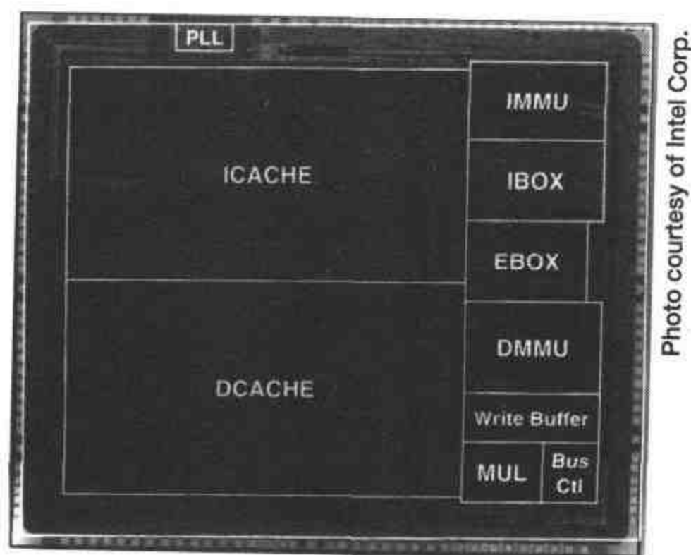
图 12.10 StrongARM 管芯照片
