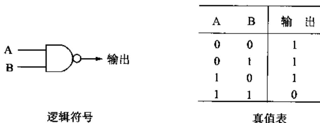
图 1.3 “与非”门逻辑符号和真值表
