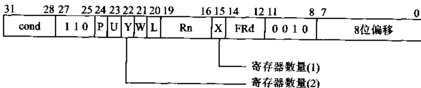
图 6.8 Load 和 Store 多浮点数的二进制编码
