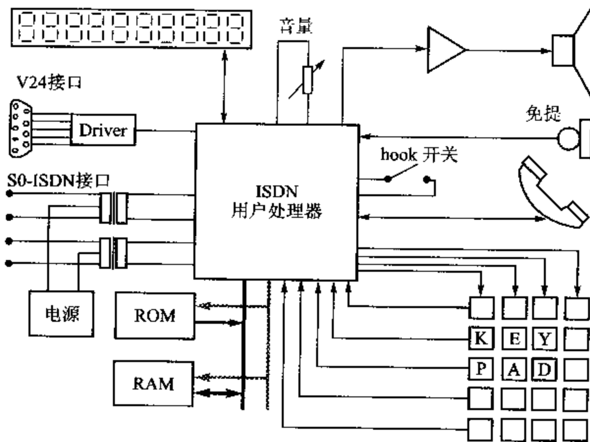
图 13.3 典型的 VIP 系统配置
