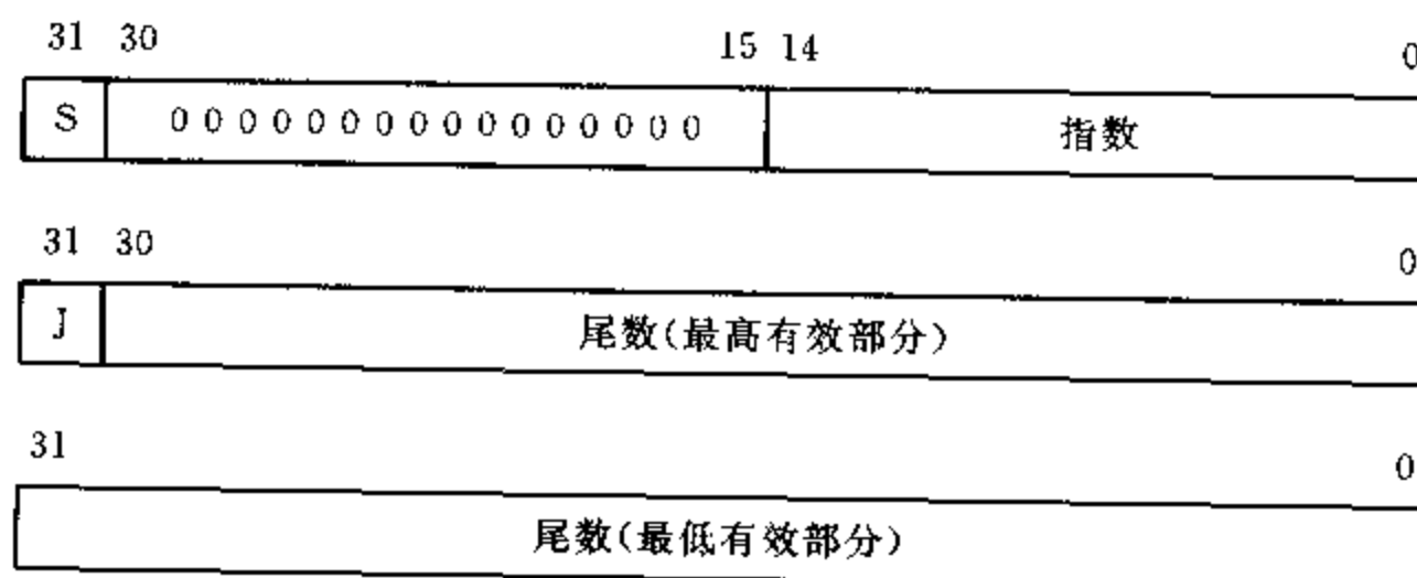
图 6.4 IEEE 754 双扩展精度浮点数格式
