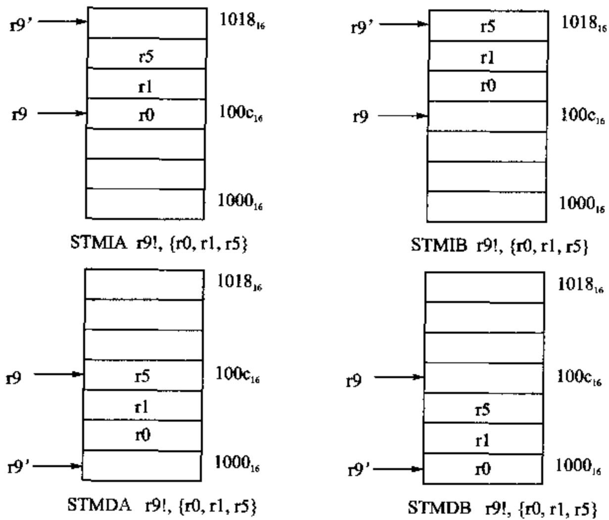
图 3.2 多寄存器传送寻址模式
