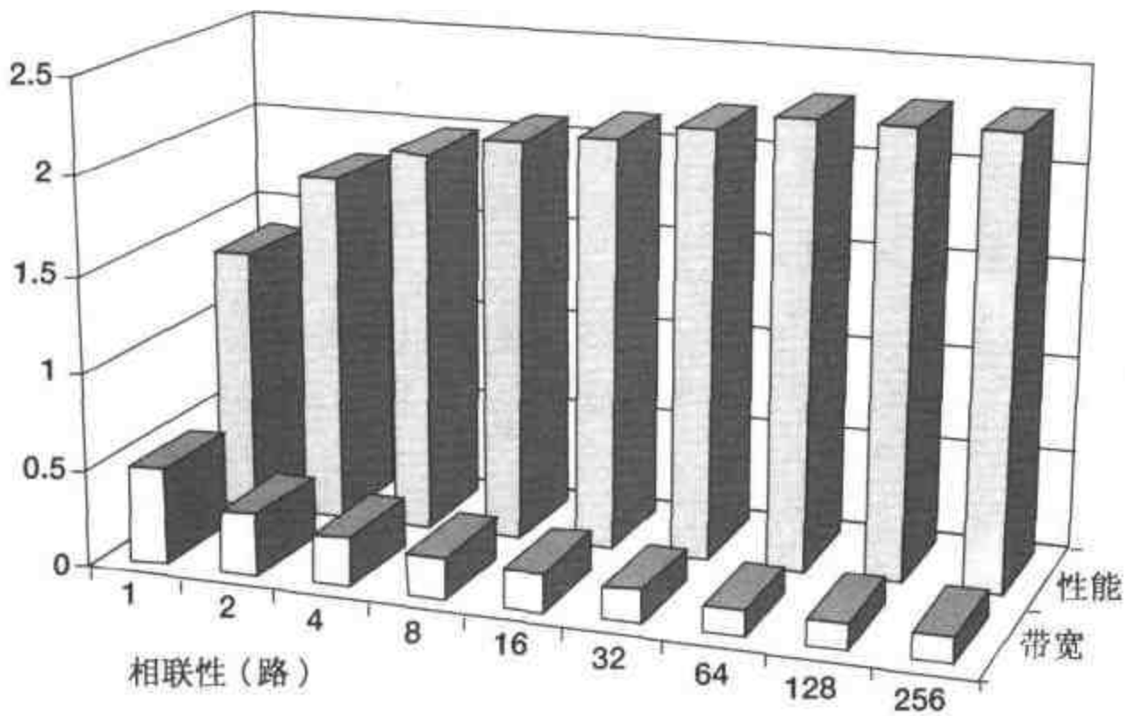
图 10.7 相联对性能及带宽需求的影响
