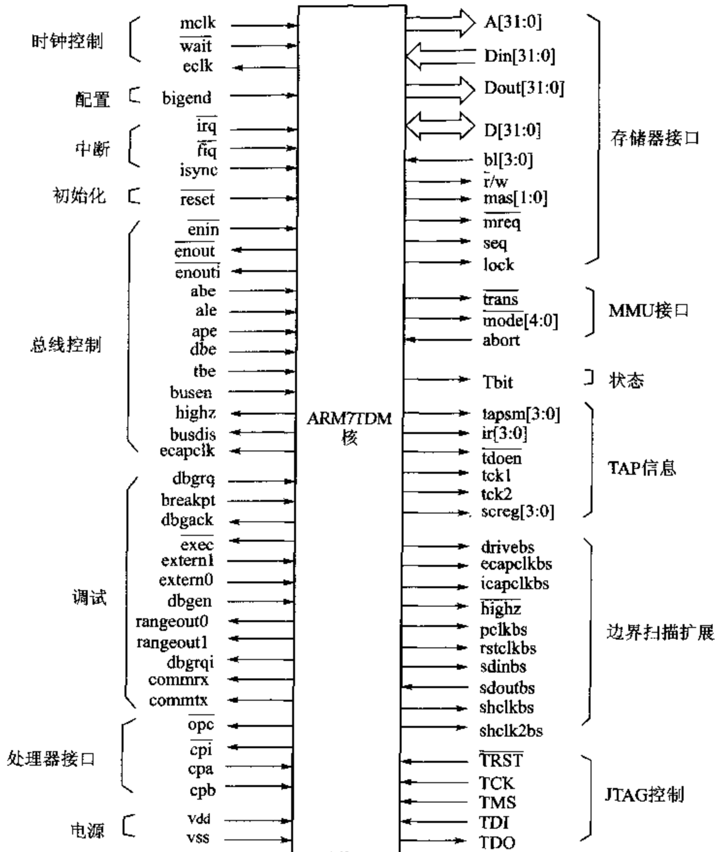
图 9.2 ARM7TDMI 核的接口信号
