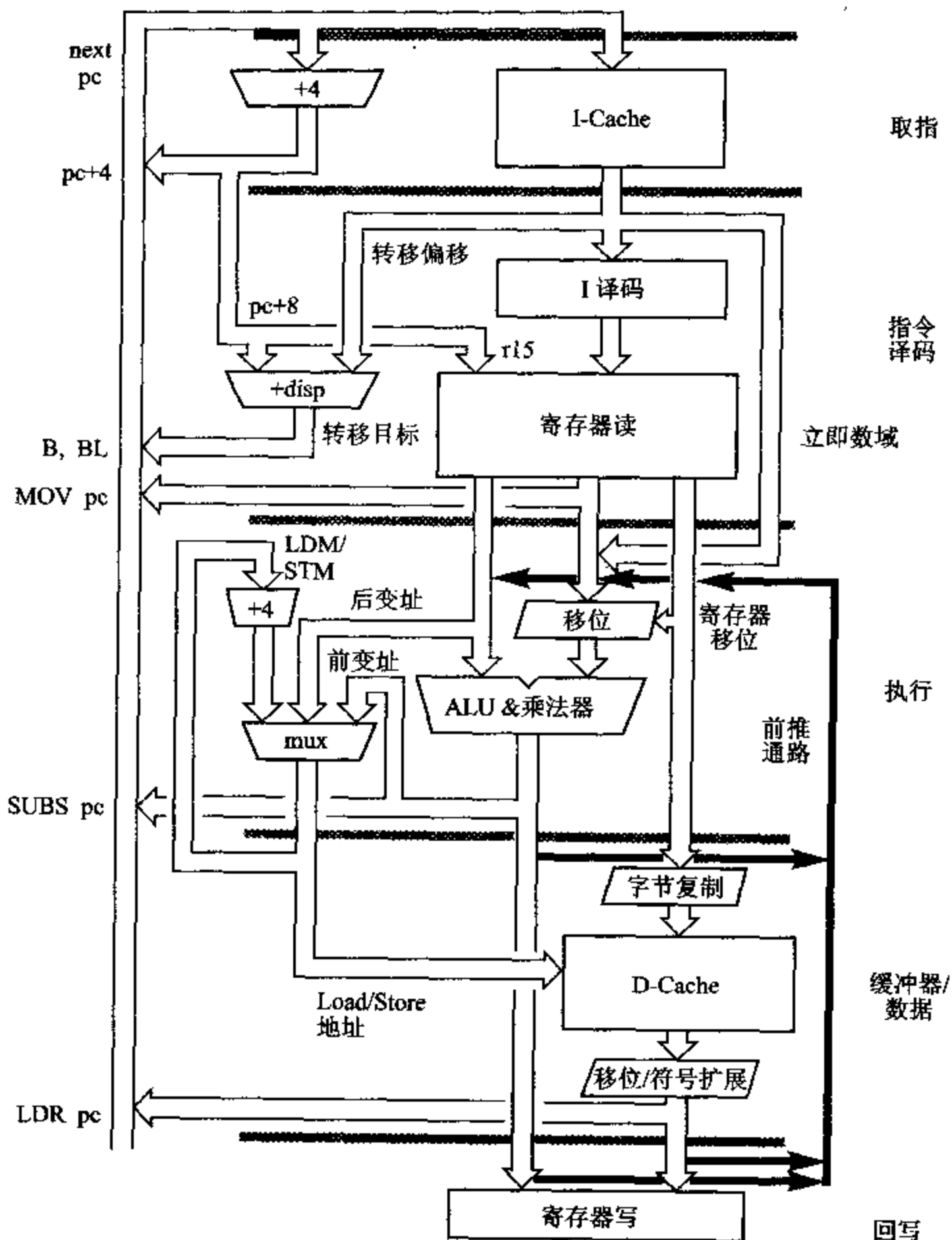
图 12.8 StrongARM 核流水线组织
