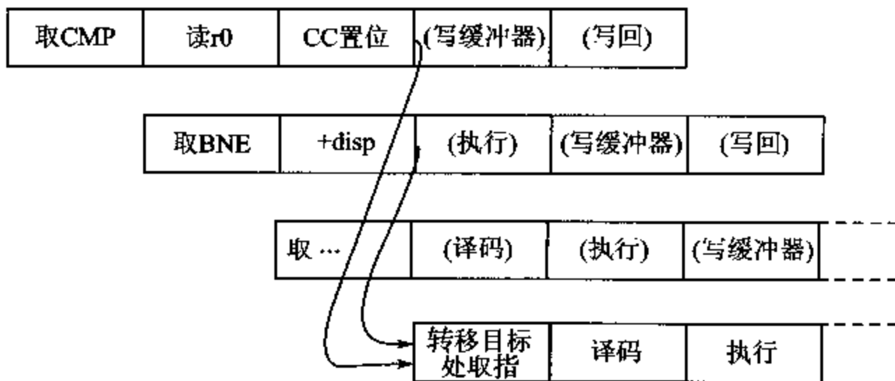
图 12.9 StrongARM 循环测试的流水线行为
