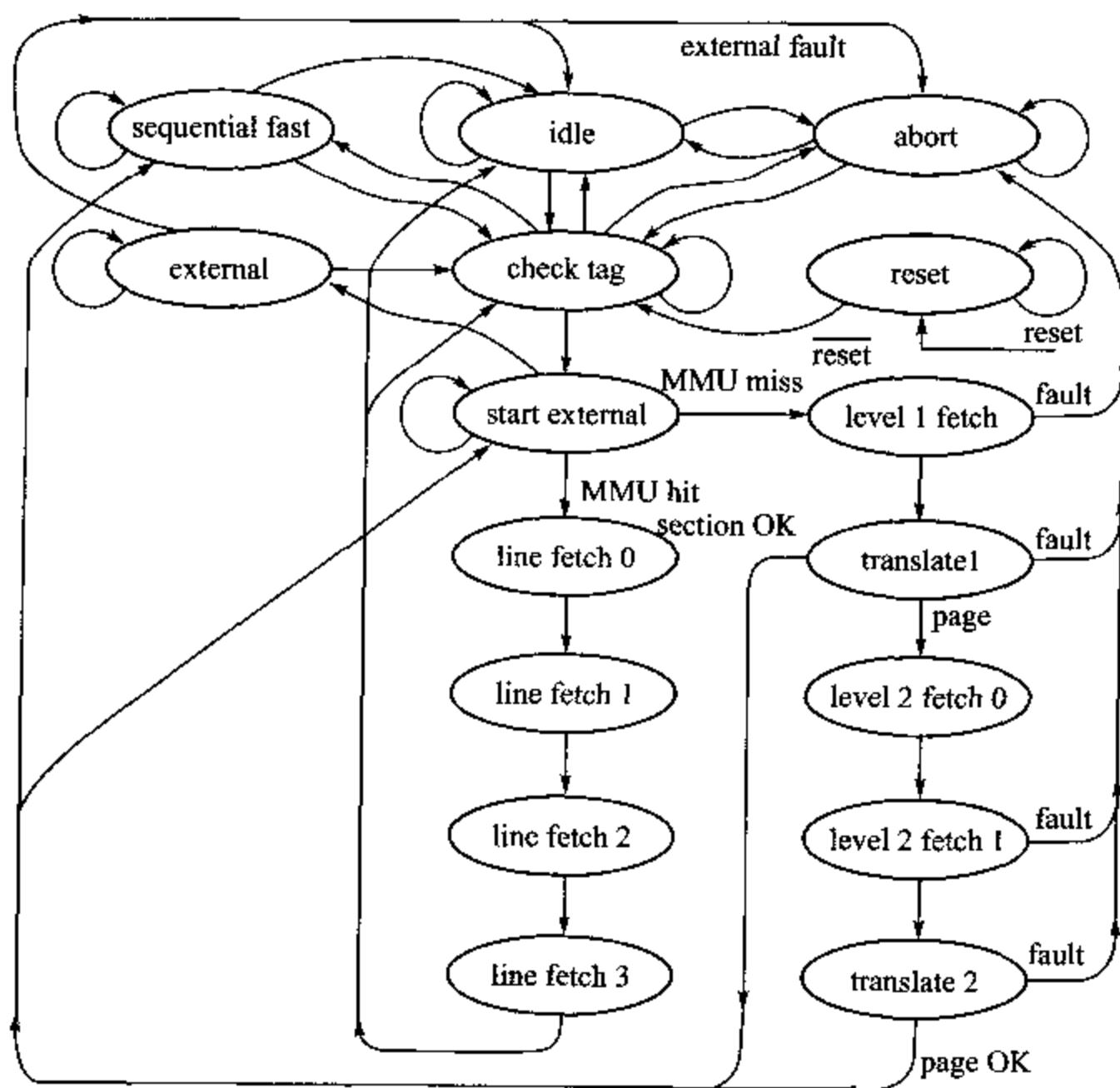
图 10.9 ARM600 Cache 控制状态机
