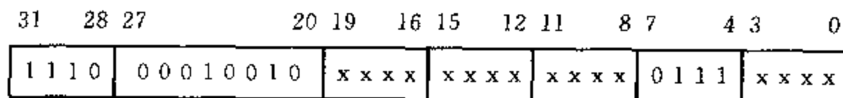
图 5.18 断点指令的二进制编码
