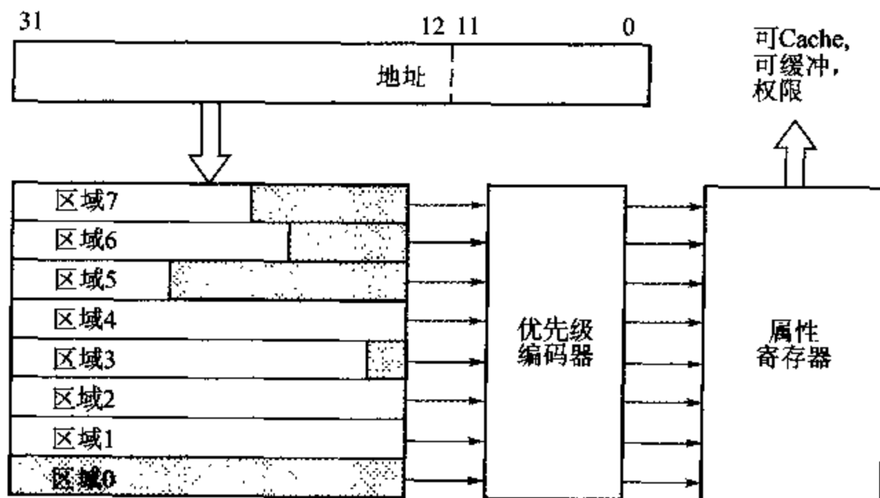
图 11.2 保护单元的组织
