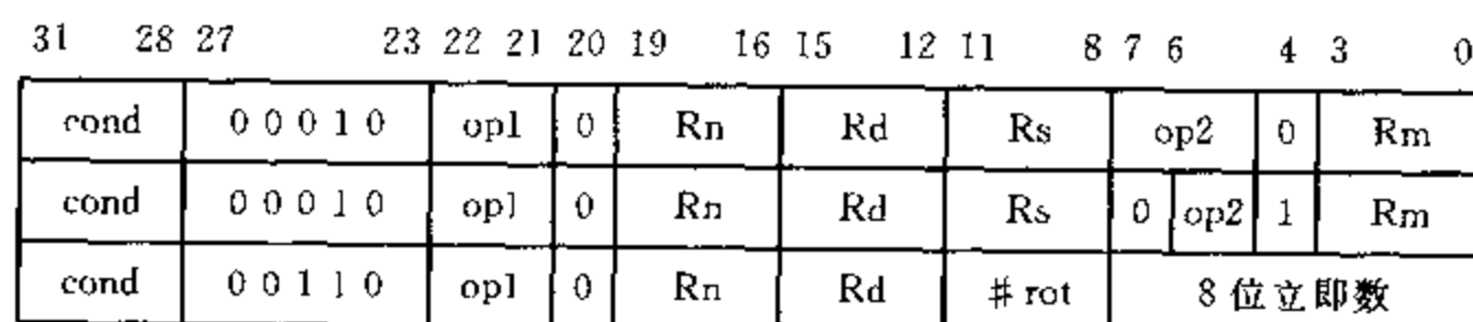
图 5.20 控制指令扩展空间
