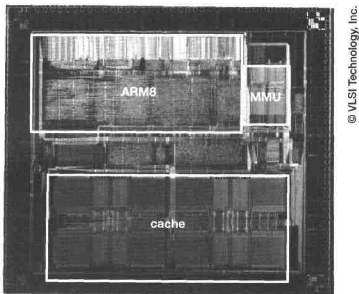
图 12.6 ARM810 管芯版图照片
