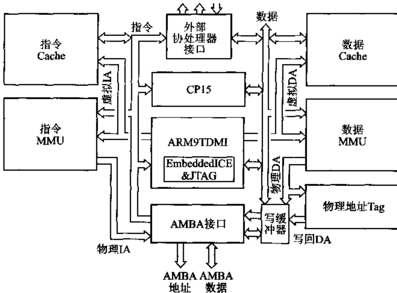
图 12.11 ARM920T 组织
