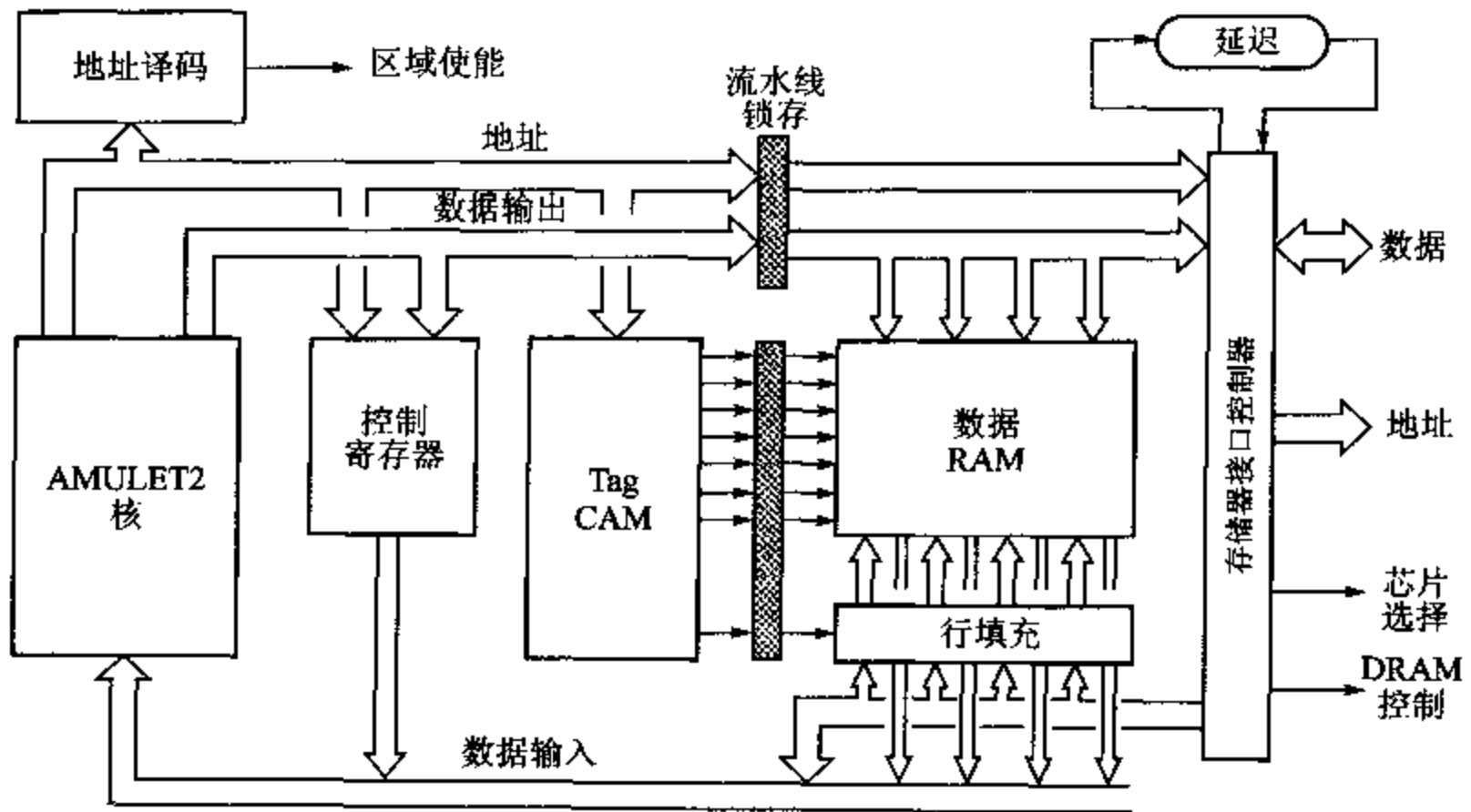
图 14.7 AMULET2e 的内部组织
