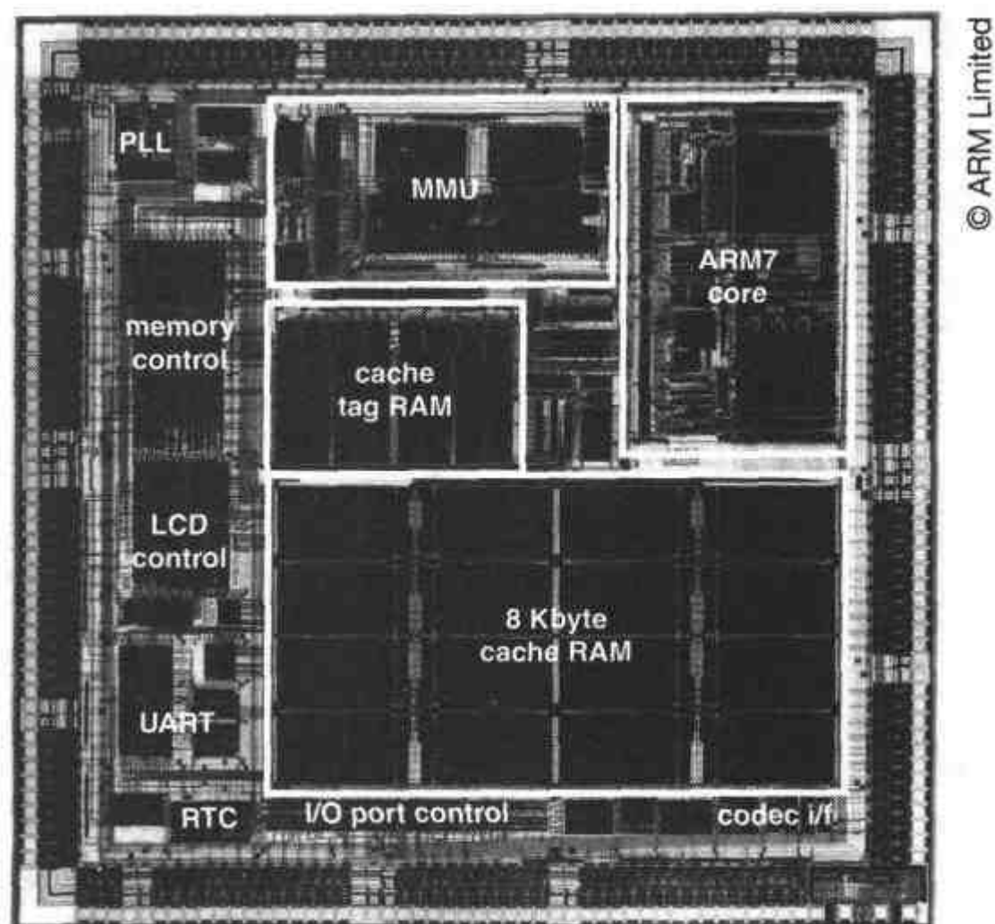
图 13.15 ARM7100 管芯图
