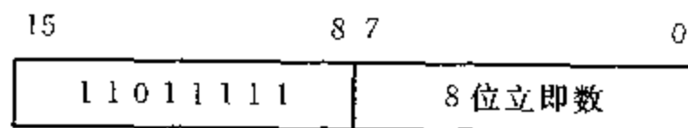
图 7.3 Thumb 软中断指令的二进制编码
