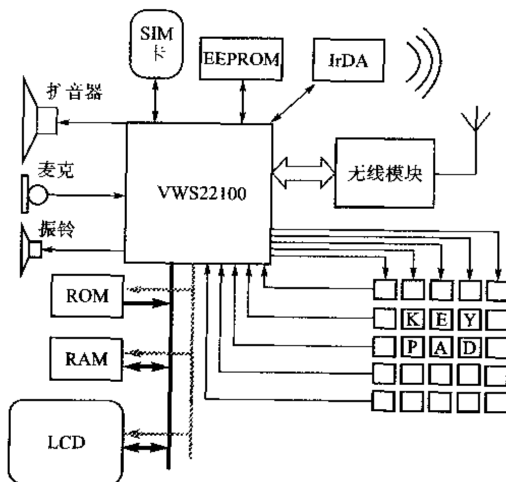
图 13.6 典型的 GSM 手机结构
