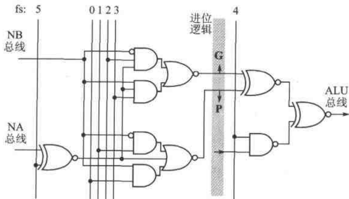
图 4.12 ARM2 的 ALU 中用于 1 位输出的逻辑
