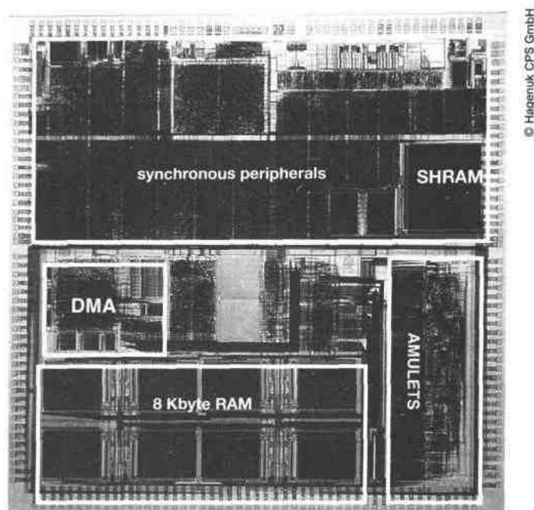
图 14.14 DRACO 的管芯图
