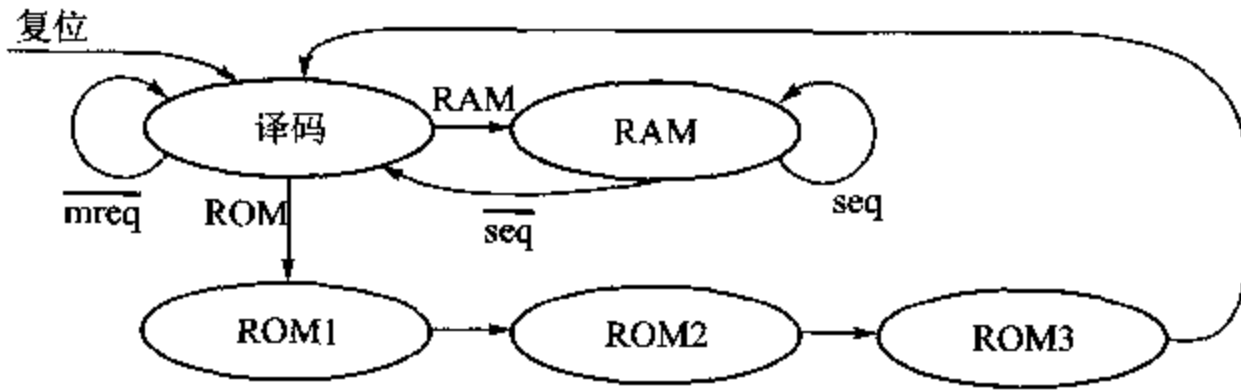
图 8.6 具有用于地址译码的等待状态的状态转换图
