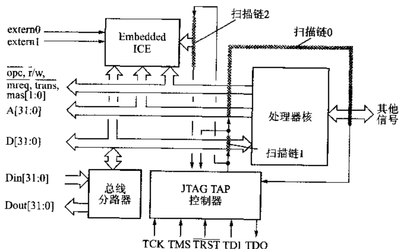
图 9.1 ARM7TDMI 的组织
