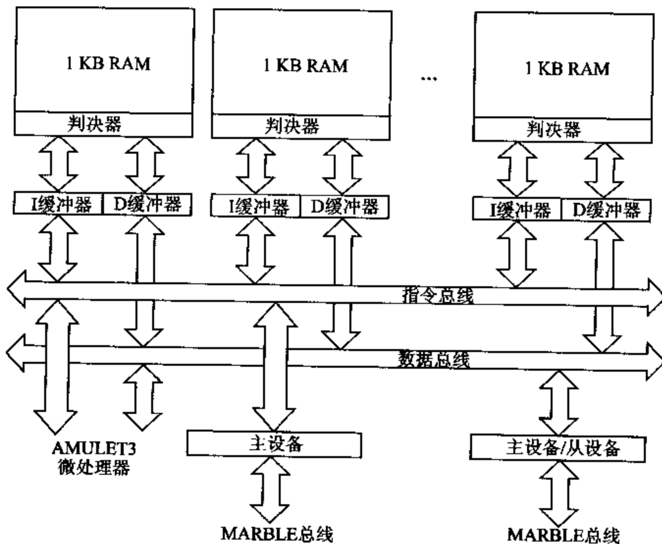
图 14.13 AMULET3H 的存储器组织
