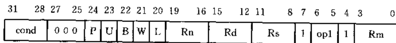
图 5.21 数据传送指令扩展空间
