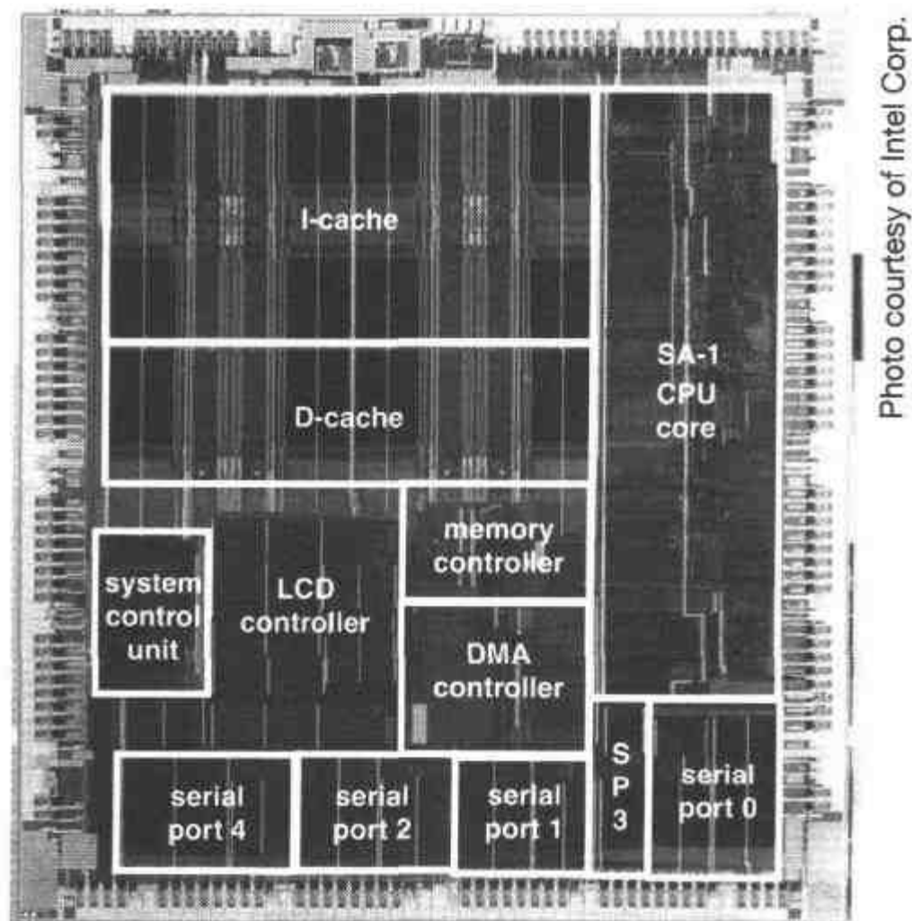
图 13.17 SA-1100 管芯图
