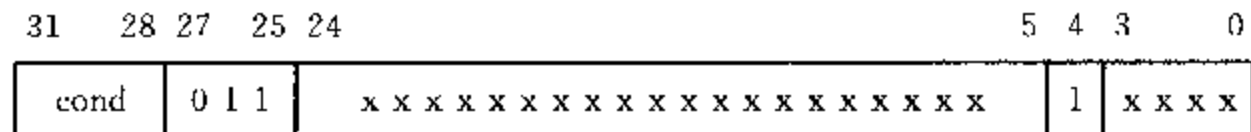
图 5.23 未定义的指令空间
