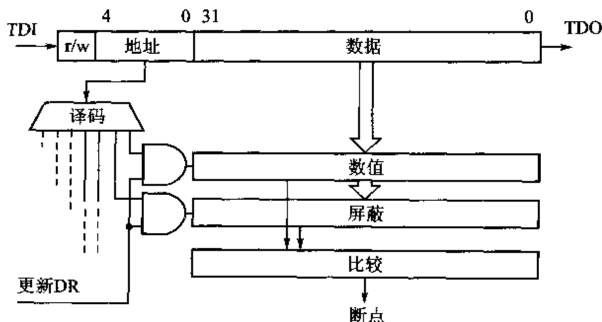
图 8.18 EmbeddedICE 寄存器读和写结构
