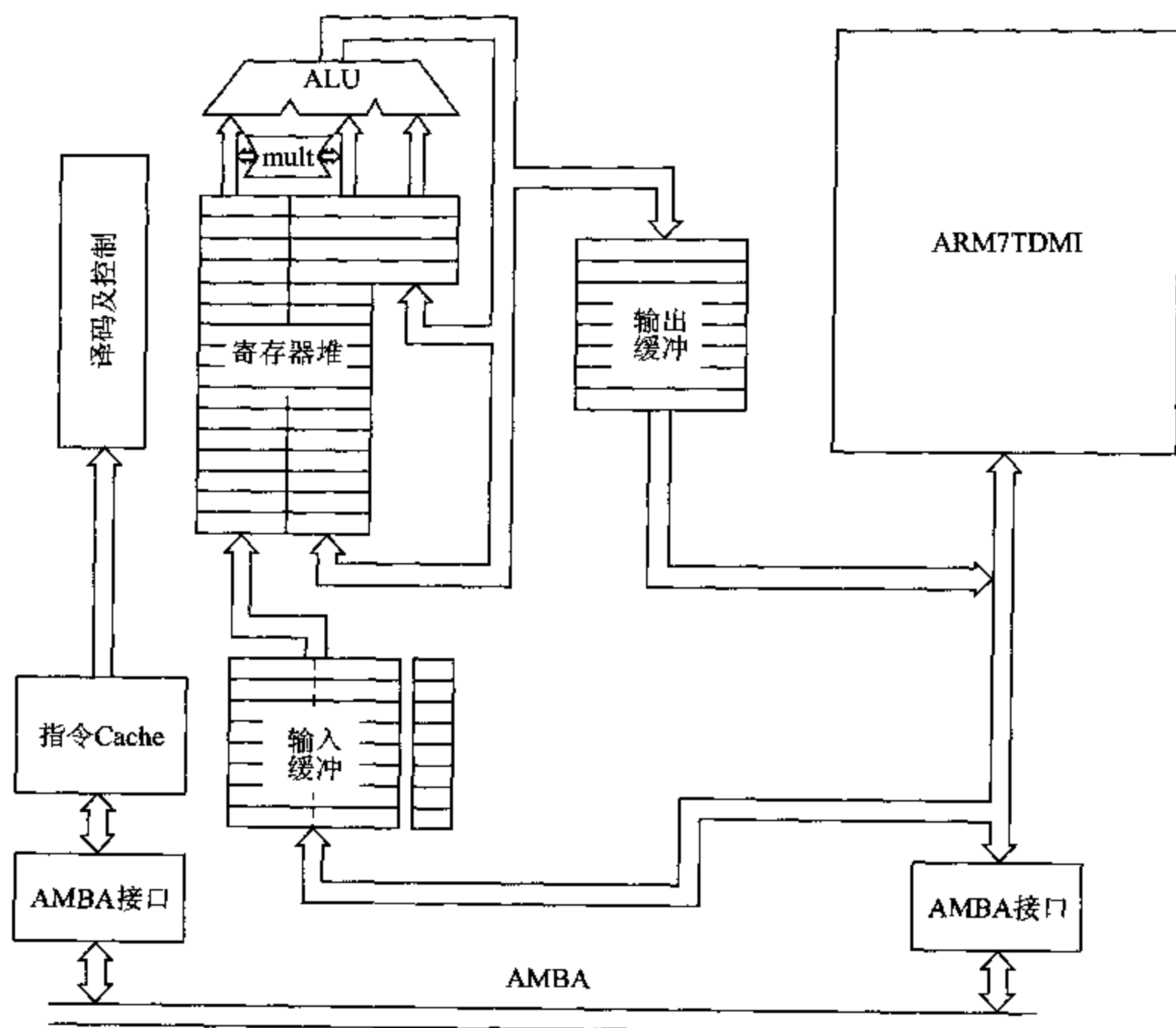
图 8.20 Piccolo 的组织
