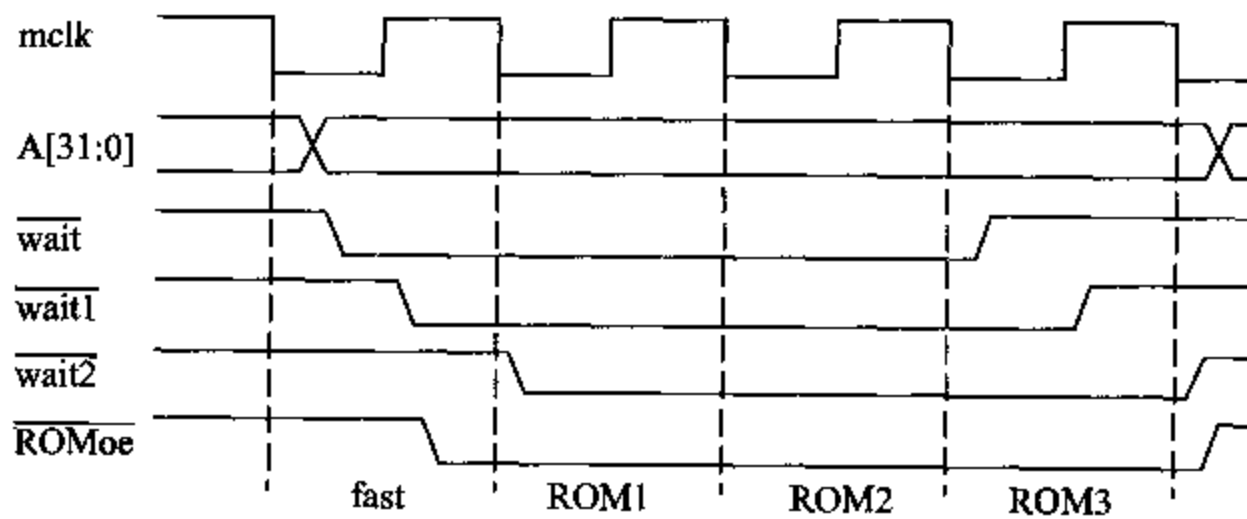
图 8.5 ROM 等待状态电路的时序
