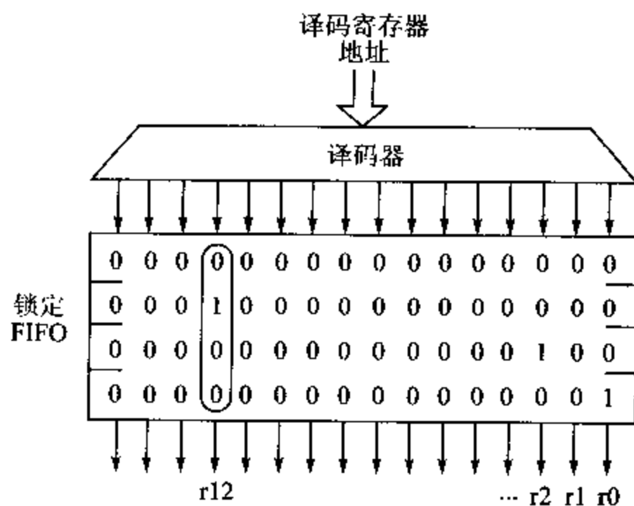
图 14.4 AMULET 中锁定寄存器的 FIFO 的组织
